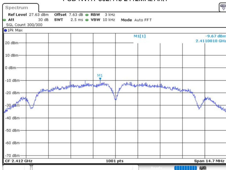
PSD NVHT 802.11b 2412MHz Ant1
