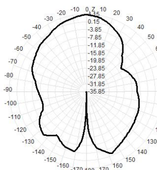
E1-Plane
