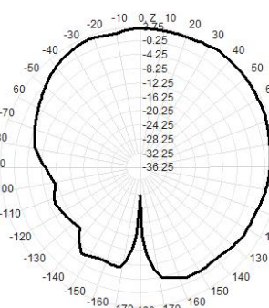
E2-Plane
