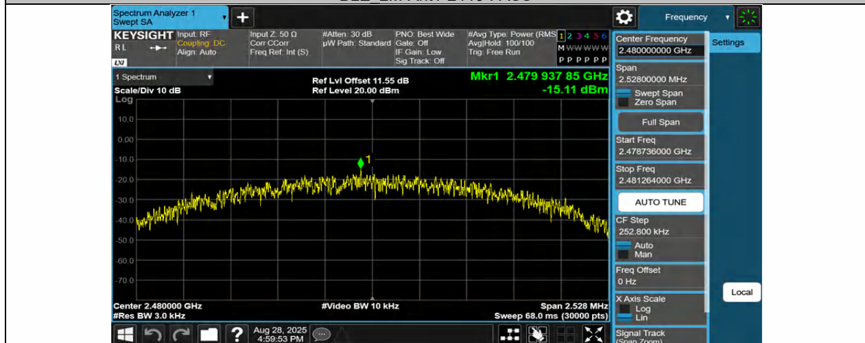
BLE 2M-Ant1-2480-PASS
