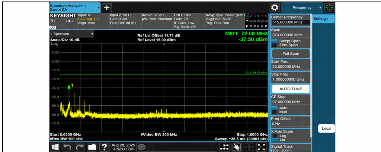
BLE_2M-Ant1-2402-30~1000-PASS
