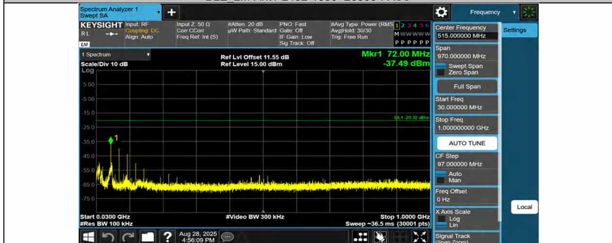
BLE_2M-Ant1-2440-30~1000-PASS
