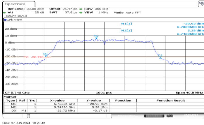
11AX20MIMO_Ant1_5745
