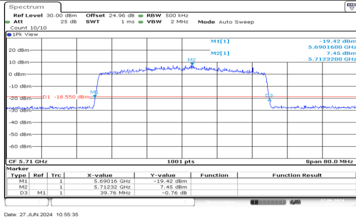
11AX40MIMO_Ant2_5710
