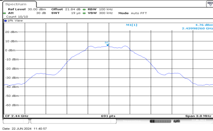
BLE 1M Ant2 2440 0~Reference
