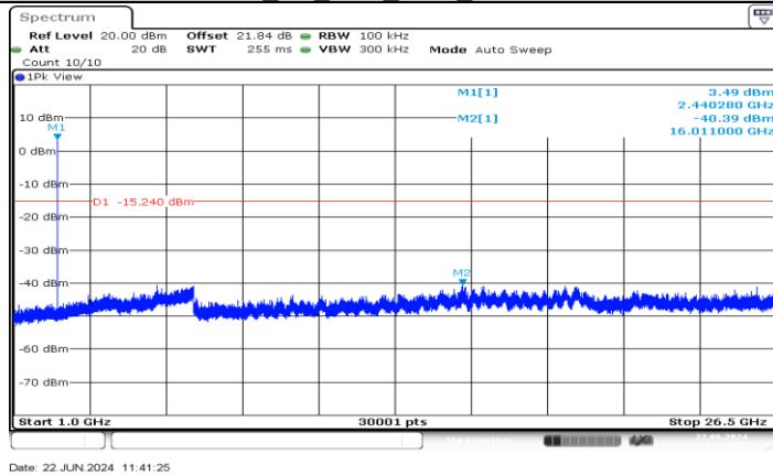
BLE 1M Ant2 2440 1000~26500
