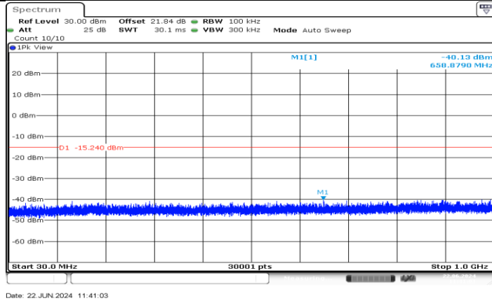
BLE 1M Ant2 2440 30~1000
