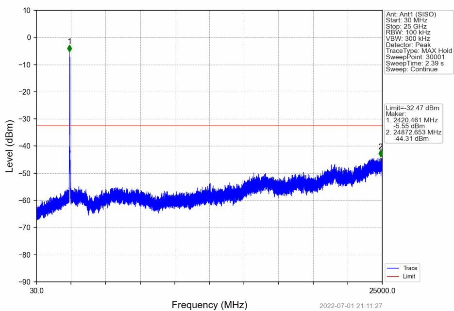
802.11n(HT40) MCH 2437MHz Ant1 (SISO) NTNV
