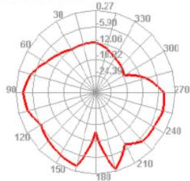
2400.000MHz E2
