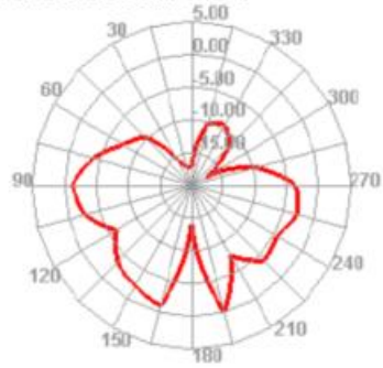
2450.000MHz E2
