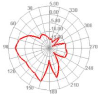
2500.000MHz E1
