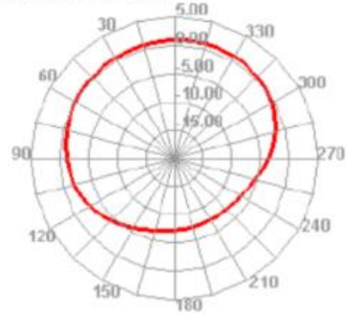
2450.000MHz H
