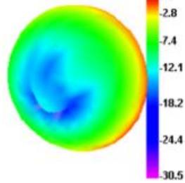
2400.000MHz
