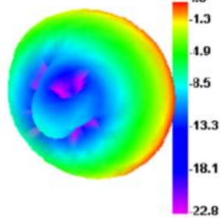
2450.000MHz
