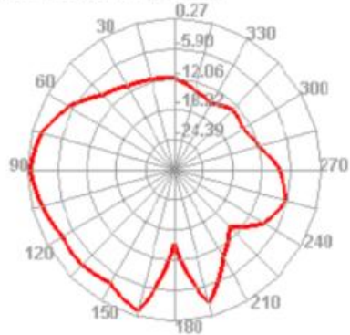
2400.000MHz E1
