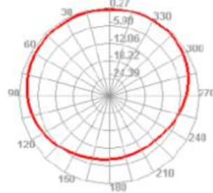
2400.000MHz H
