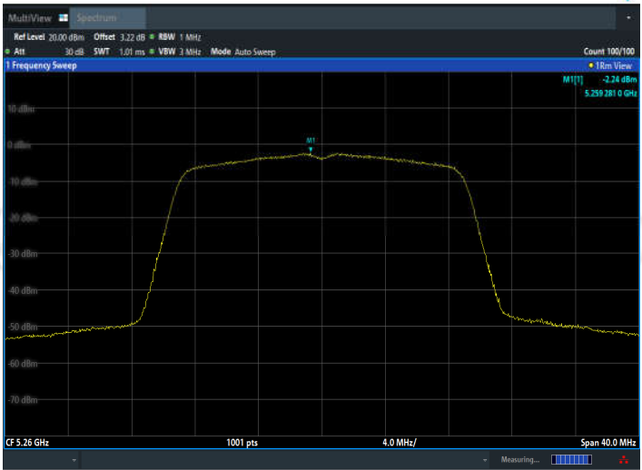
11AC20MIMO_Ant2_5260
