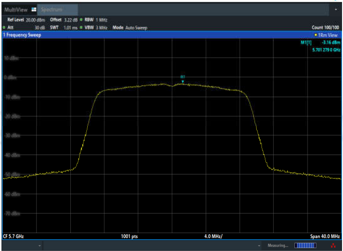
11AC20MIMO_Ant2_5700
