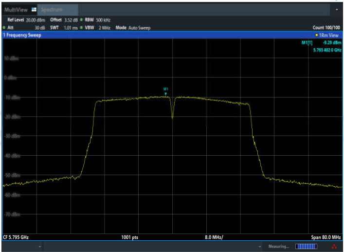
11AC40MIMO_Ant2_5795
