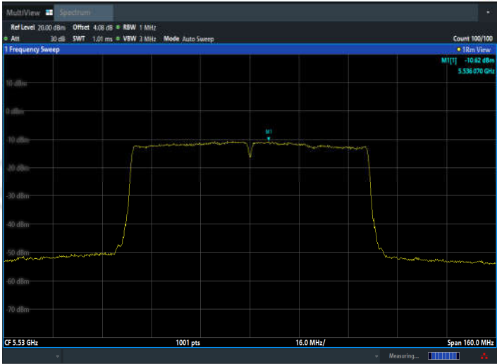
11AC80MIMO_Ant2_5530
