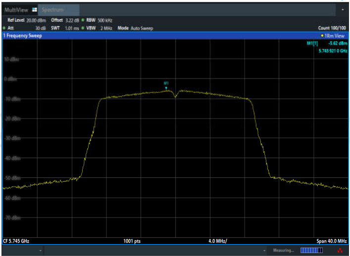
11N20MIMO_Ant2_5745
