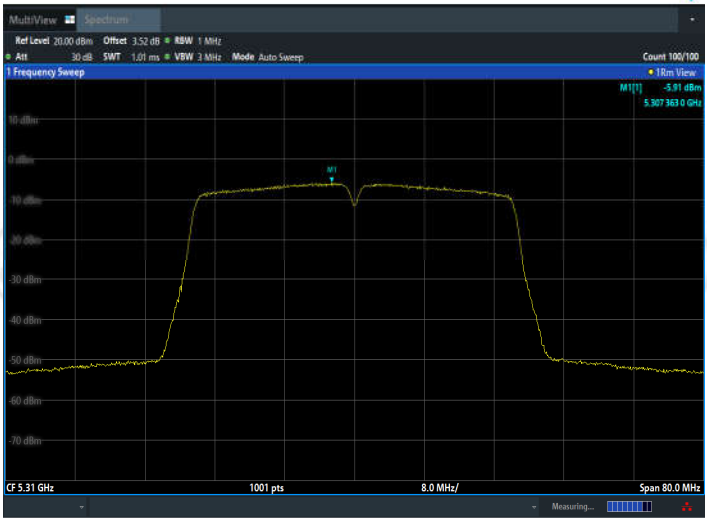
11AC40MIMO_Ant2_5310
