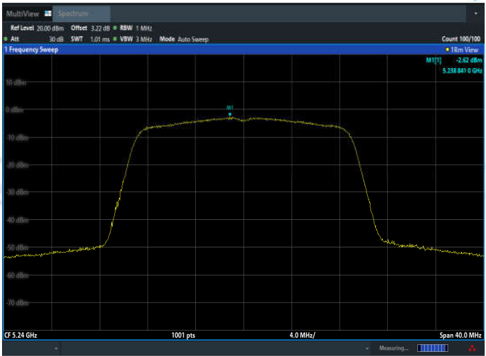
11N20MIMO_Ant2_5240
