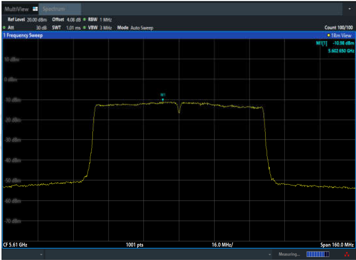
11AC80MIMO_Ant2_5610
