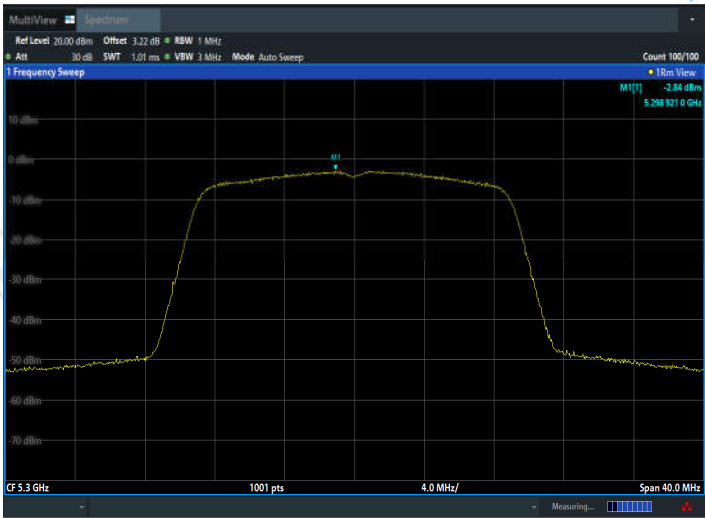
11N20MIMO_Ant2_5300
