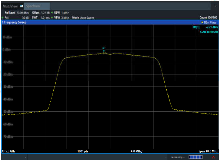
11AC20MIMO_Ant2_5300
