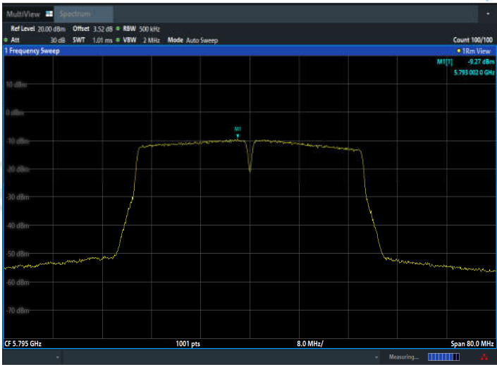
11N40MIMO_Ant2_5795
