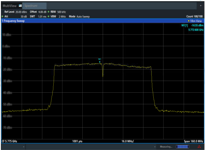
11AC80MIMO_Ant2_5775
