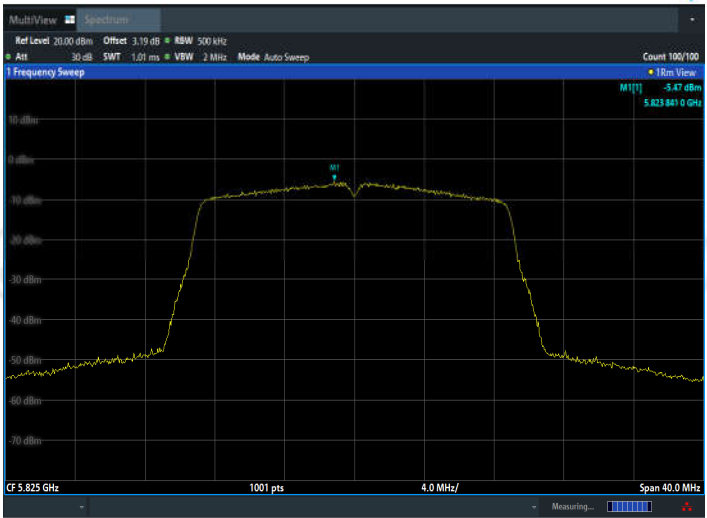
11N20MIMO_Ant2_5825
