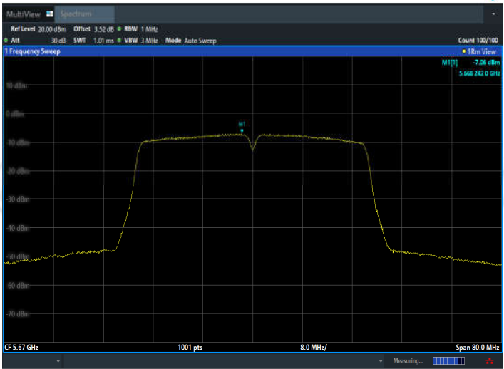
11AC40MIMO_Ant2_5670
