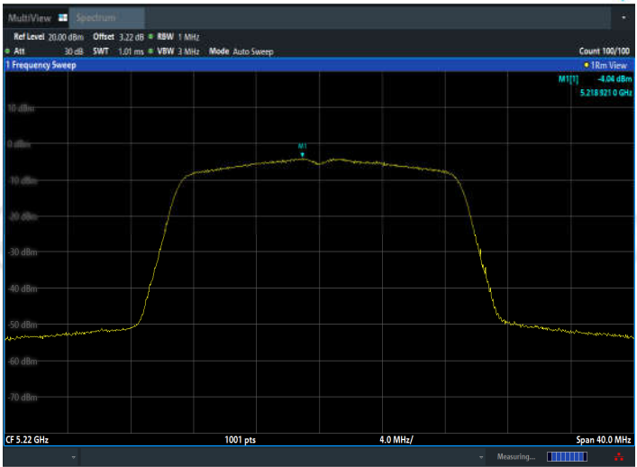
11N20MIMO_Ant2_5220
