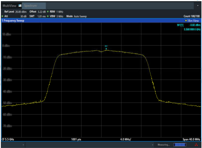
11N20MIMO_Ant2_5500
