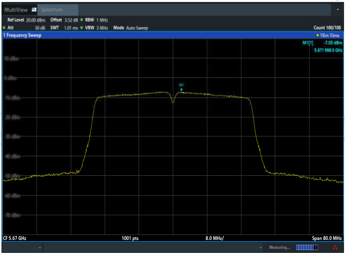
11N40MIMO_Ant2_5670
