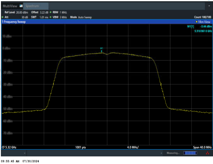
11N20MIMO_Ant2_5320
