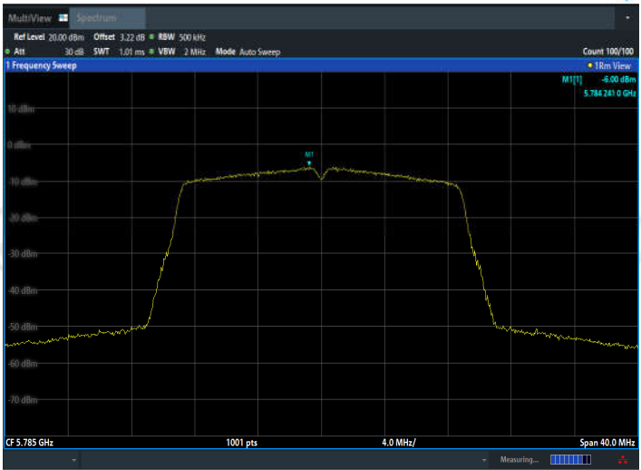
11N20MIMO_Ant2_5785
