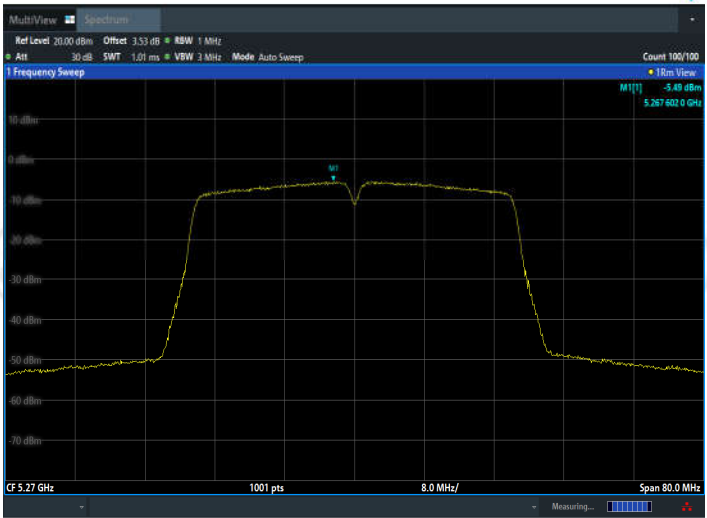
11N40MIMO_Ant2_5270
