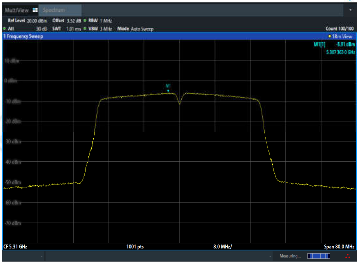
11N40MIMO_Ant2_5310
