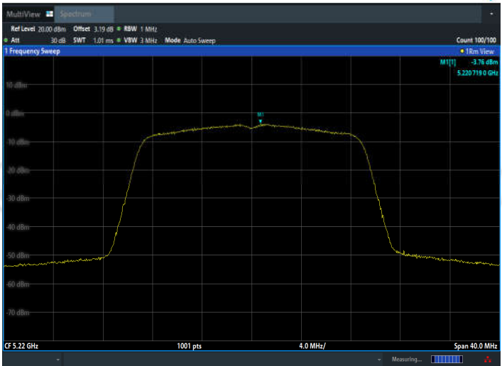
11AC20MIMO_Ant2_5220
