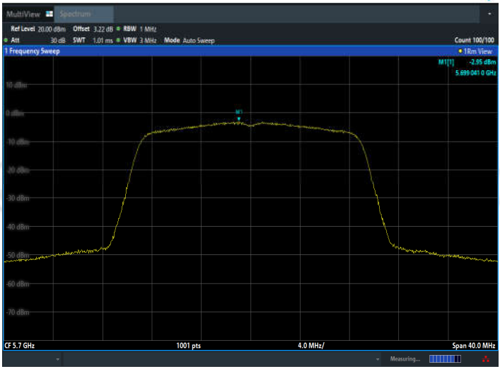
11N20MIMO_Ant2_5700
