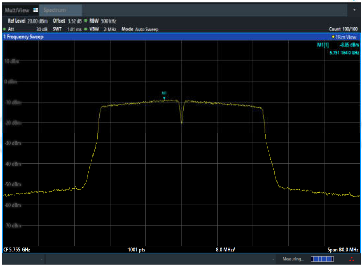
11N40MIMO_Ant2_5755
