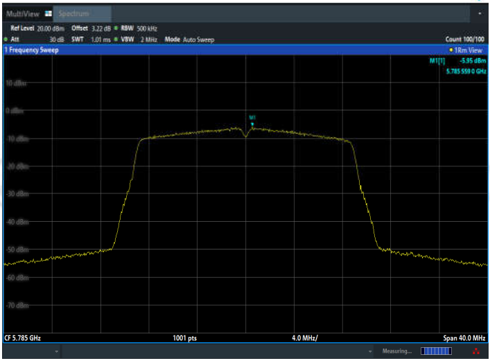
11AC20MIMO_Ant2_5785
