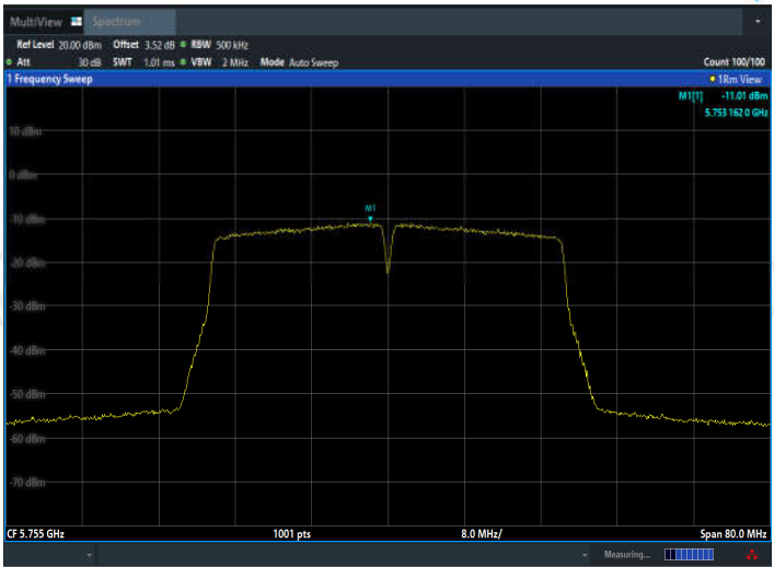
11AC40MIMO_Ant2_5755
