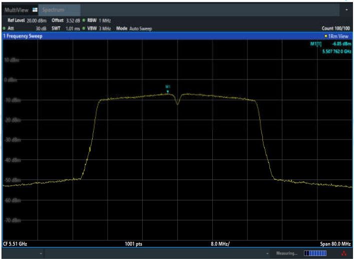
11AC40MIMO_Ant2_5510
