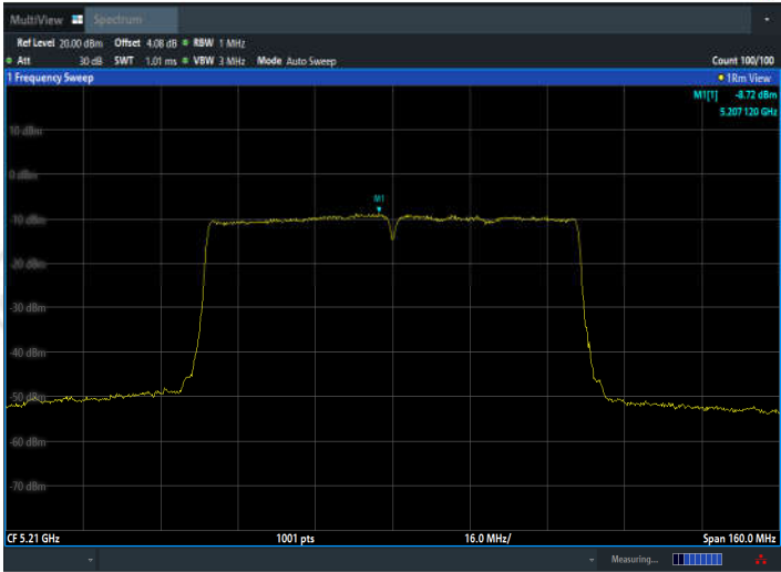
11AC80SISO_Ant2_5210
