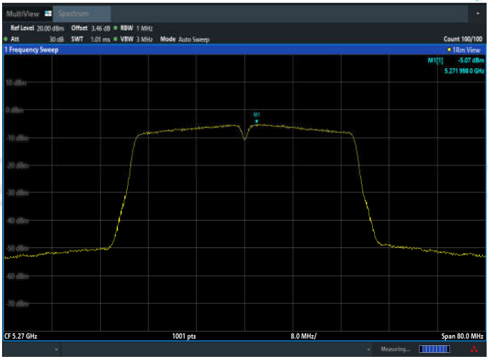
11AC40MIMO_Ant2_5270
