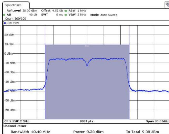
11AC40MIMO_Ant2_5550
