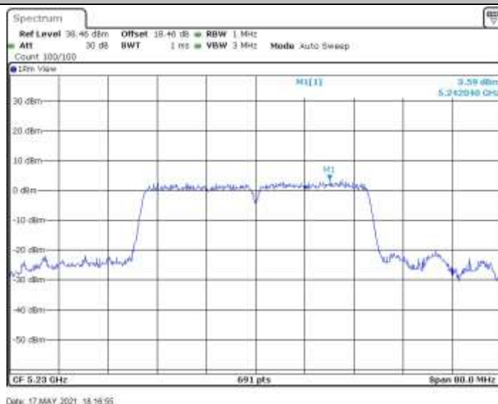
11N40SISO_Ant2_5230
