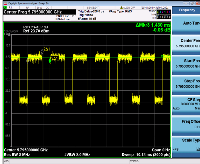
11N40SISO_Ant2_5795
