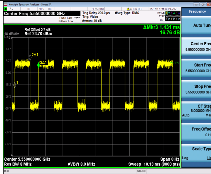
11N40SISO_Ant2_5550
