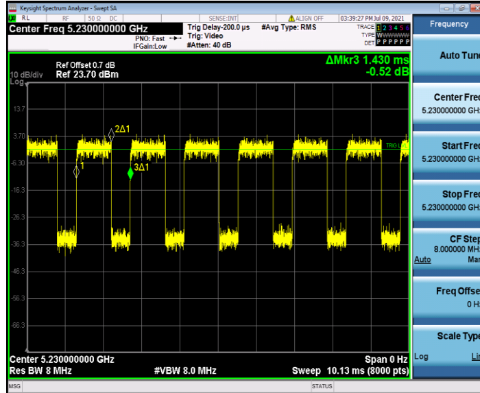
11N40SISO_Ant2_5230
