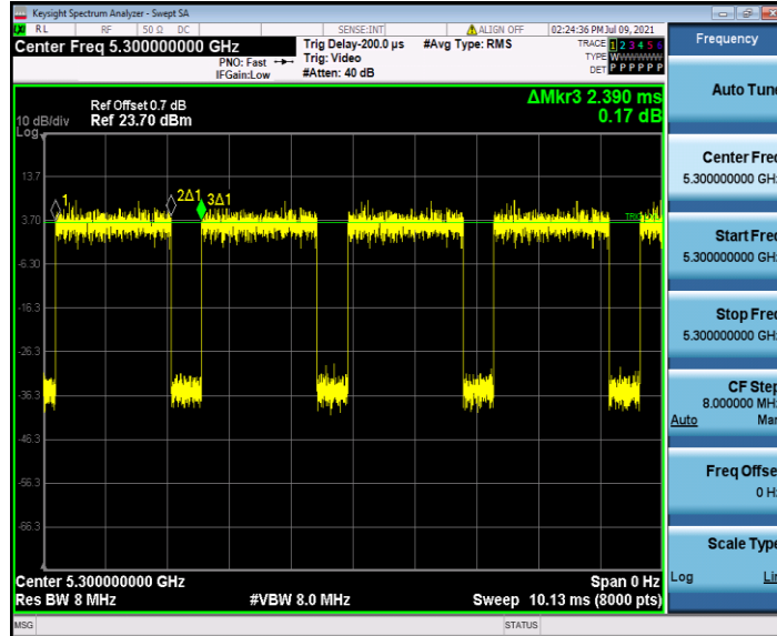
11N20SISO_Ant2_5300
