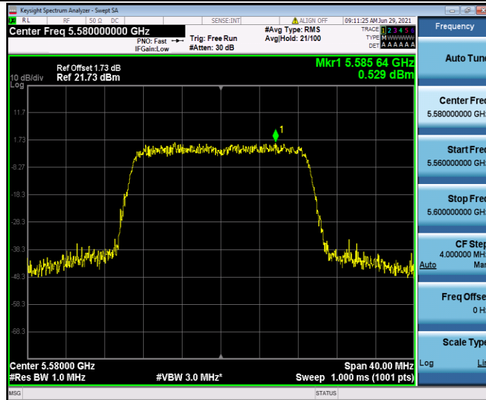
11N20SISO_Ant2_5580
