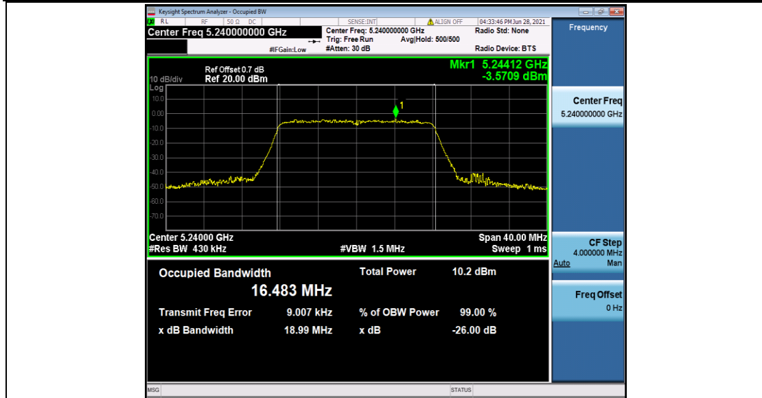
11A_Ant2_5240
