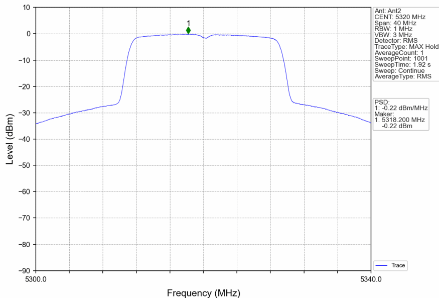
802.11n(HT20)_HCH_5320MHz_MIMO_NTNV
