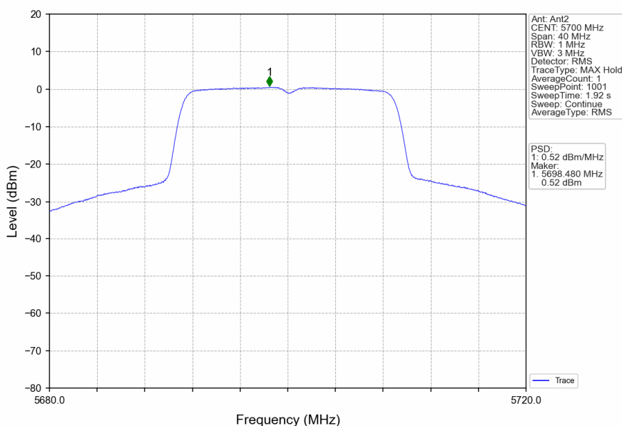
802.11n(HT20)_HCH_5700MHz_Ant2_NTNV
