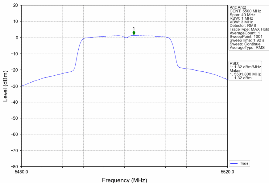
802.11n(HT20)_LCH_5500MHz_Ant2_NTNV
