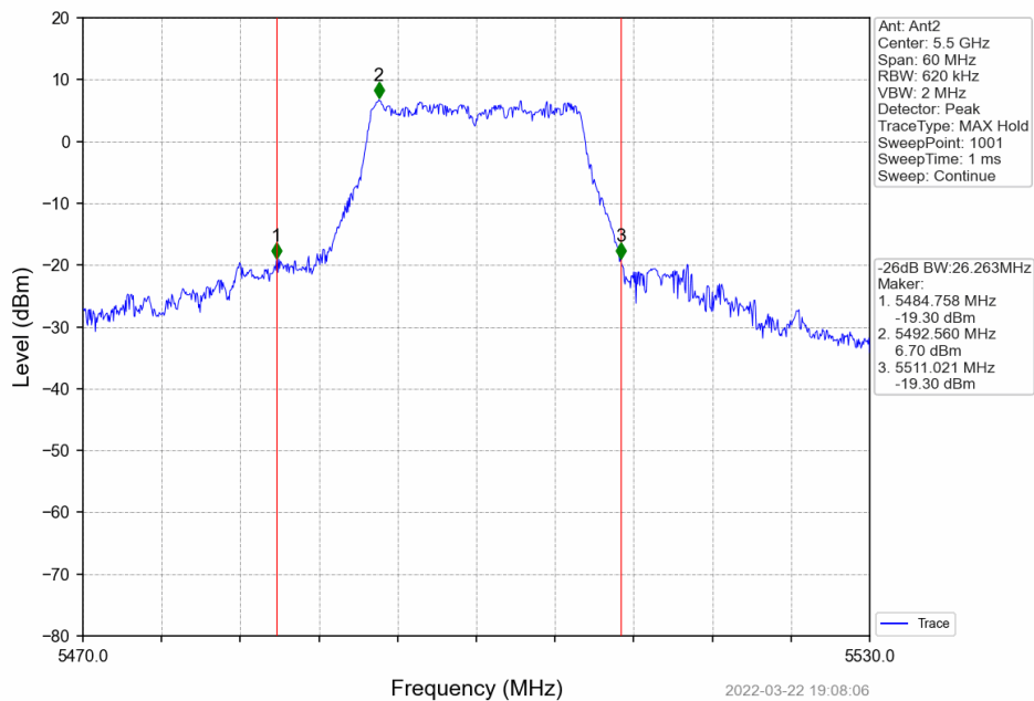
802.11a LCH 5500MHz Ant2 NTV
