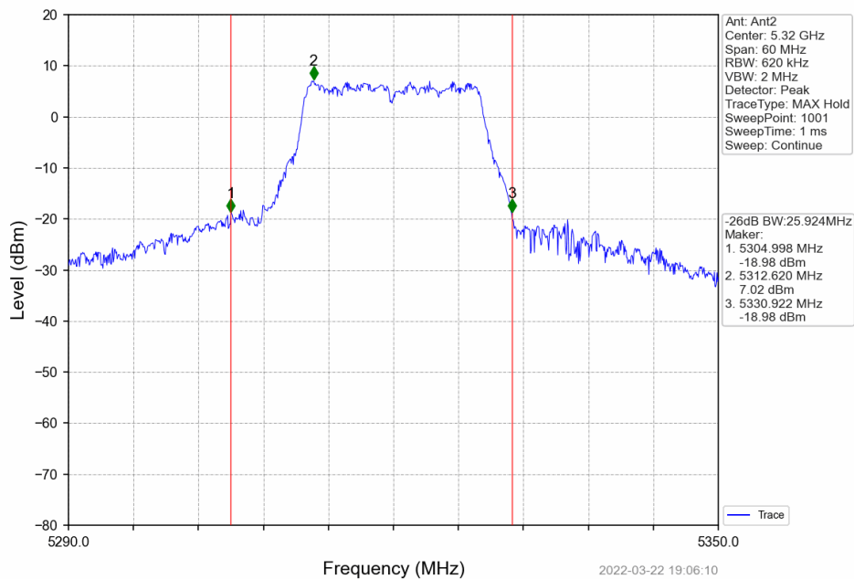
802.11a HCH 5320MHz Ant2 NTV
