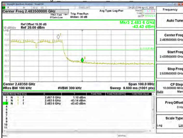
Band Edge 802.11n 40MHz Chain1 2452MHz
