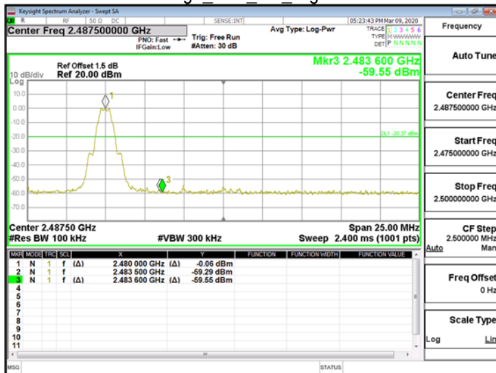
1M/Band Edge BLE 1M HighCH39-2480
