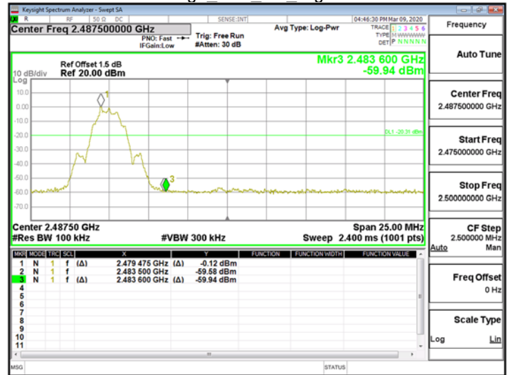
2M/Band Edge BLE 2M HighCH39-2480
