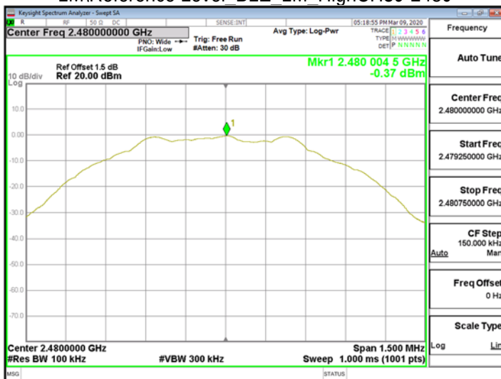
1MReference Level BLE 1M HighCH39-2480
