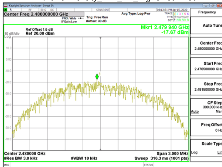
2M Power Density BLE 2M HighCH39-2480
