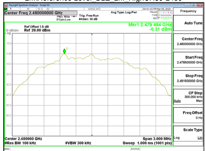
2MReference Level BLE 2M HighCH39-2480
