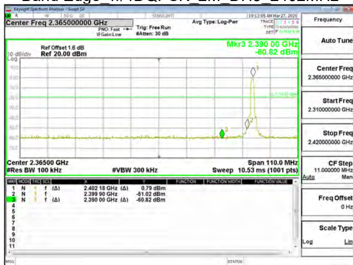
Band Edge \pi/4 DQPSK 2M DH5 2402MHz
