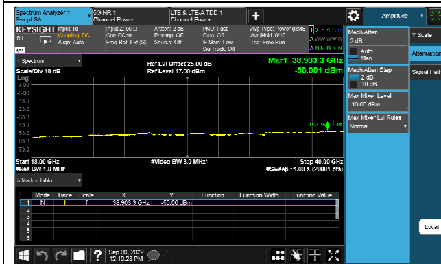
QPSK_3555MHz+3685MHz+3695MHz
