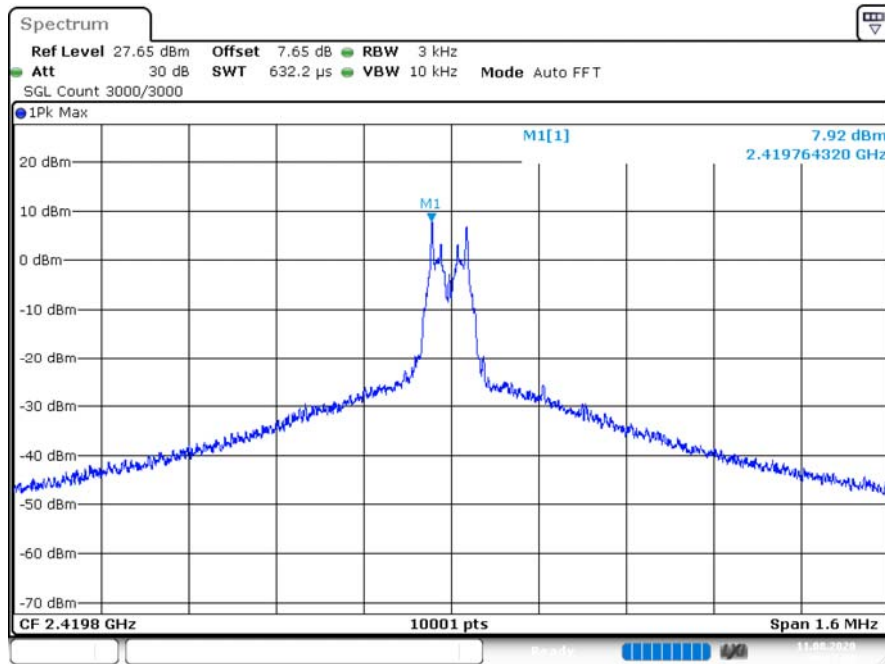
PSD NVNT GFSK 2419.8MHz Ant1
