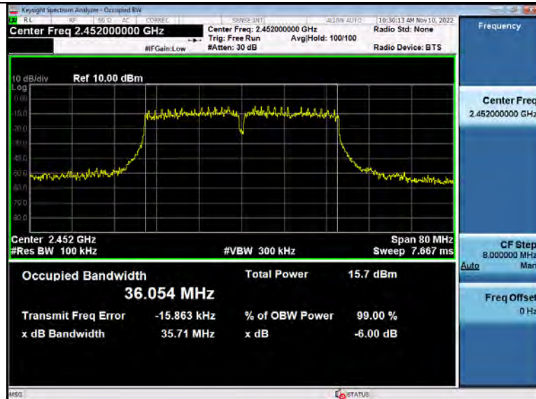
-6dB Bandwidth 2_4GWiFi 2452_00_ANT1
