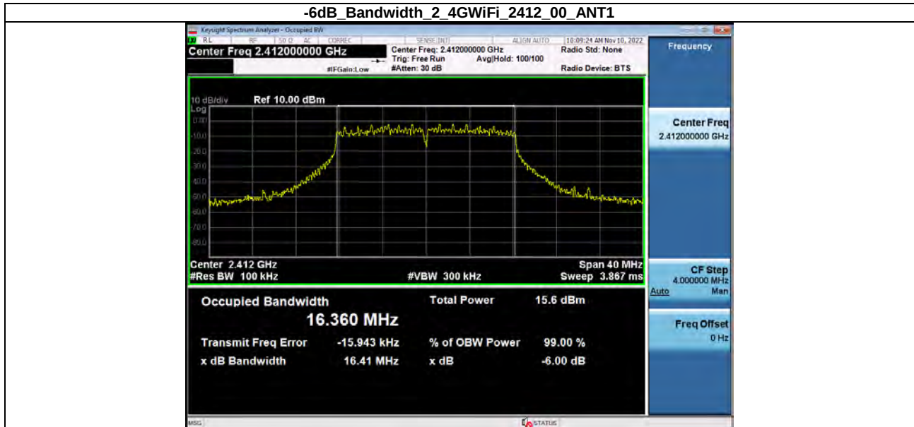
-6dB_Bandwidth_2_4GWiFi_2412_00_ANT1
