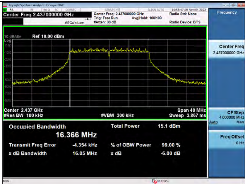
-6dB_Bandwidth_2_4GWiFi_2437_00-ANT1
