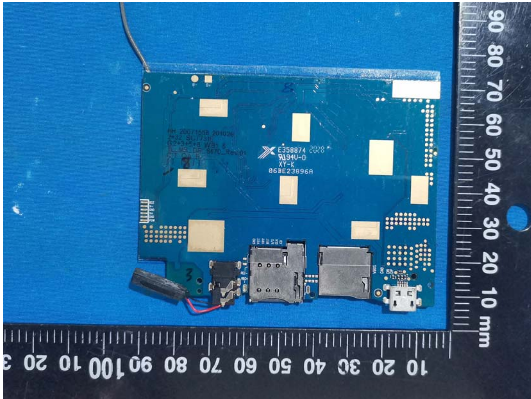
GSM/WCDMA Antenna
