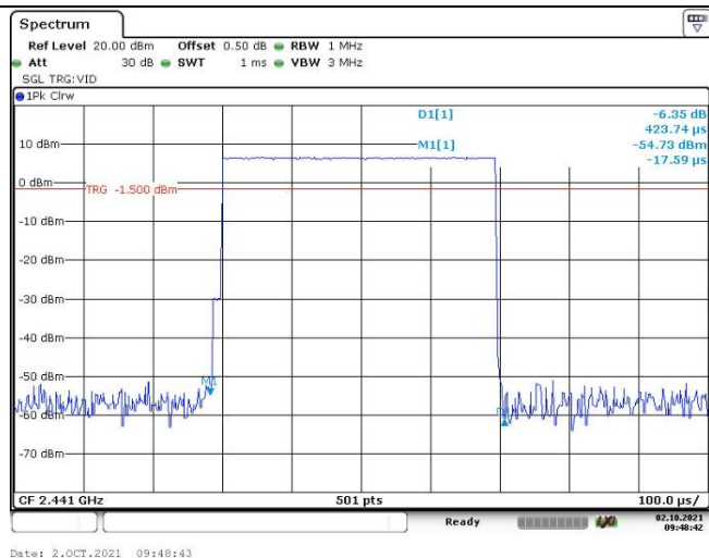
EDR Mode ( \pi/4 -DQPSK)
