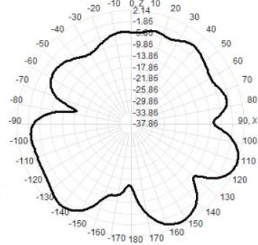
5150.0MHz Total(E1-XZ), Max= -1.81dBi
