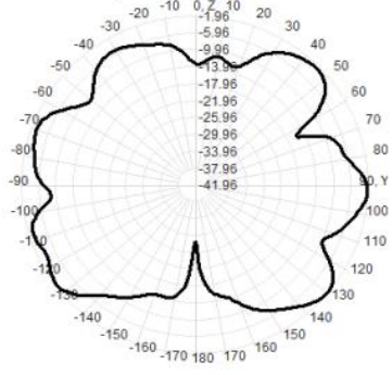
5350.0MHz Total(E2-YZ), Max= -2.34dBi
