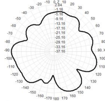
2450.0MHz Total(E1-XZ), Max= 1.19dBi
