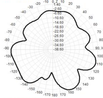
2500.0MHz Total(E1-XZ), Max= 1.85dBi
