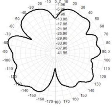
5350.0MHz Total(E1-XZ), Max= -2.30dBi
