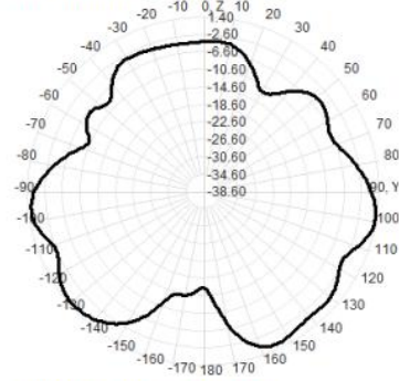
2500.0MHz Total(E2-YZ), Max= 0.80dBi
