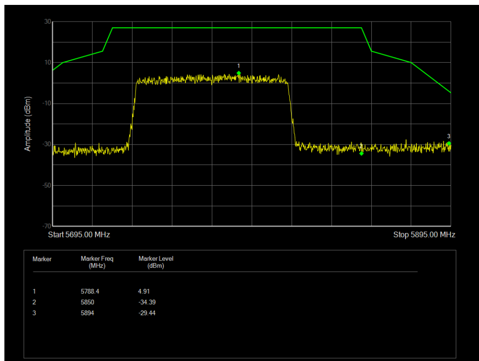
Band Edge NVNT 802.11ac80 5775MHz High Ant 4
