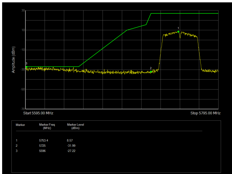
Band Edge NVNT 802.11n(HT40) 5755MHz Low Ant 4
