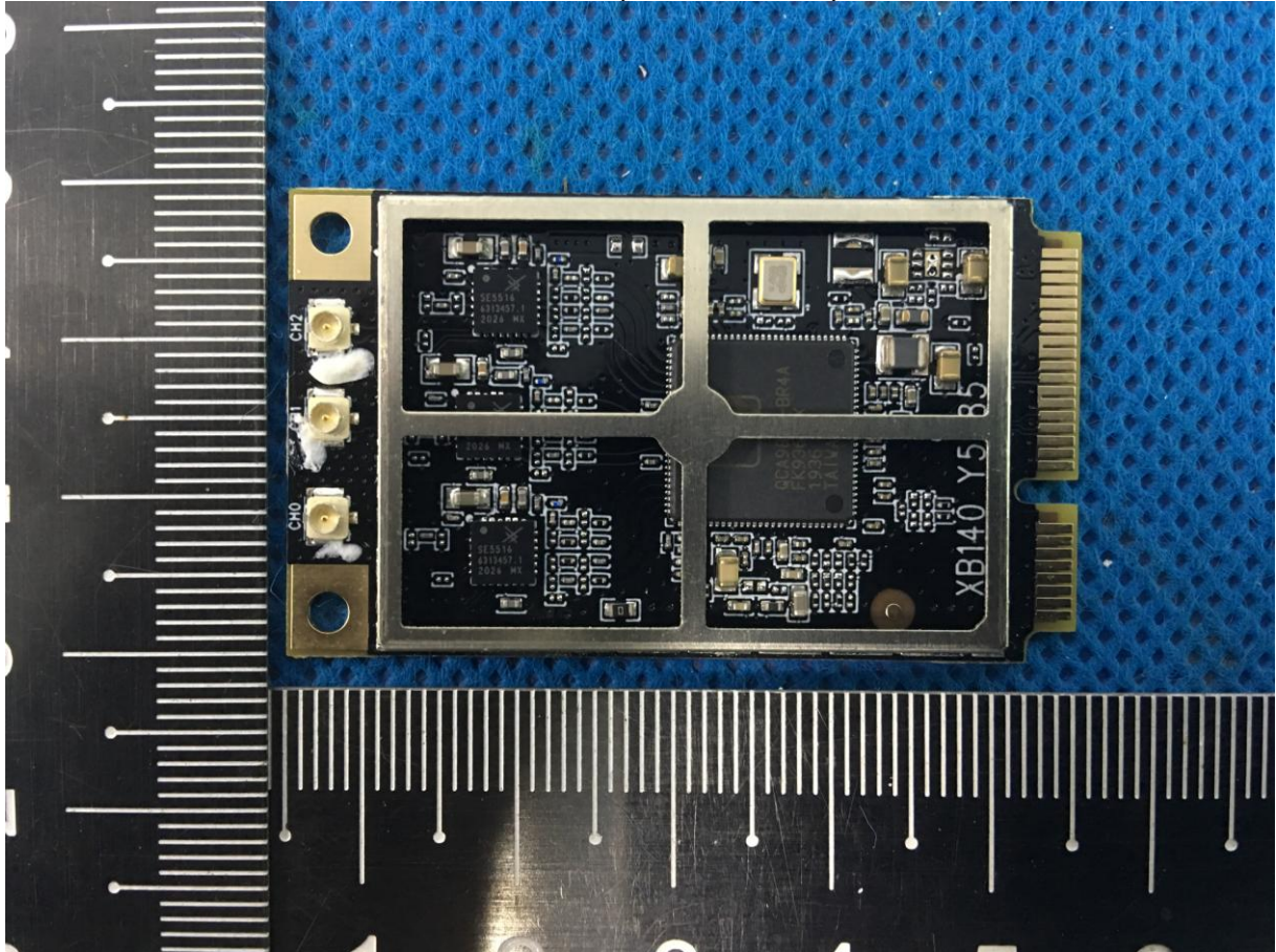
Photo14 (LTE1 Module)
