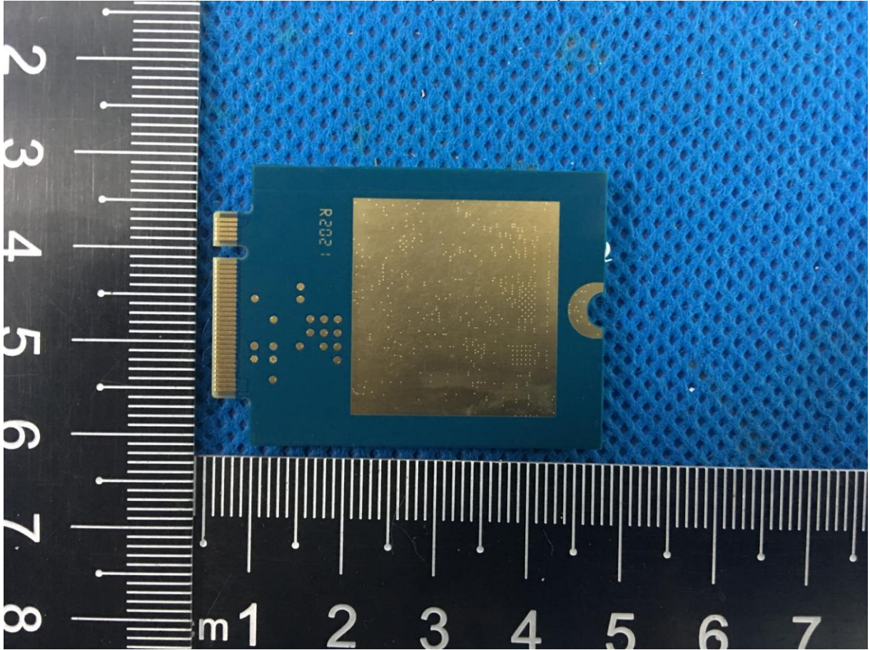
Photo16 (LTE2 Module)
