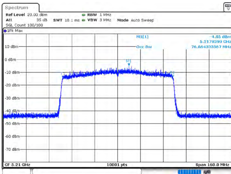
OBW NVNT 802.11ax80 5210MHz Ant 1
