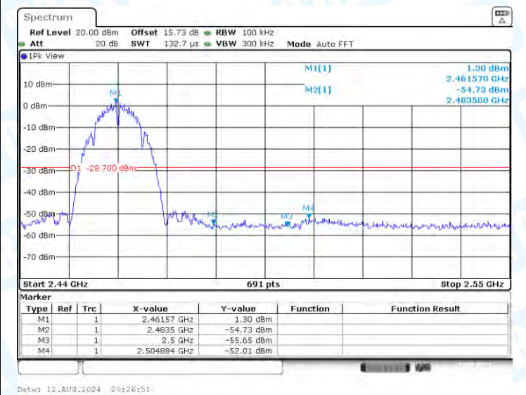
11B-Ant2-2462-PASS
