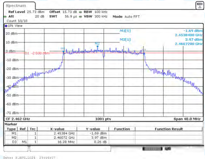
11G-CDD-Ant2-2462-PASS
