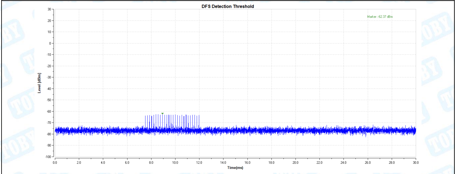
11AX40-5270-Type2-PASS
