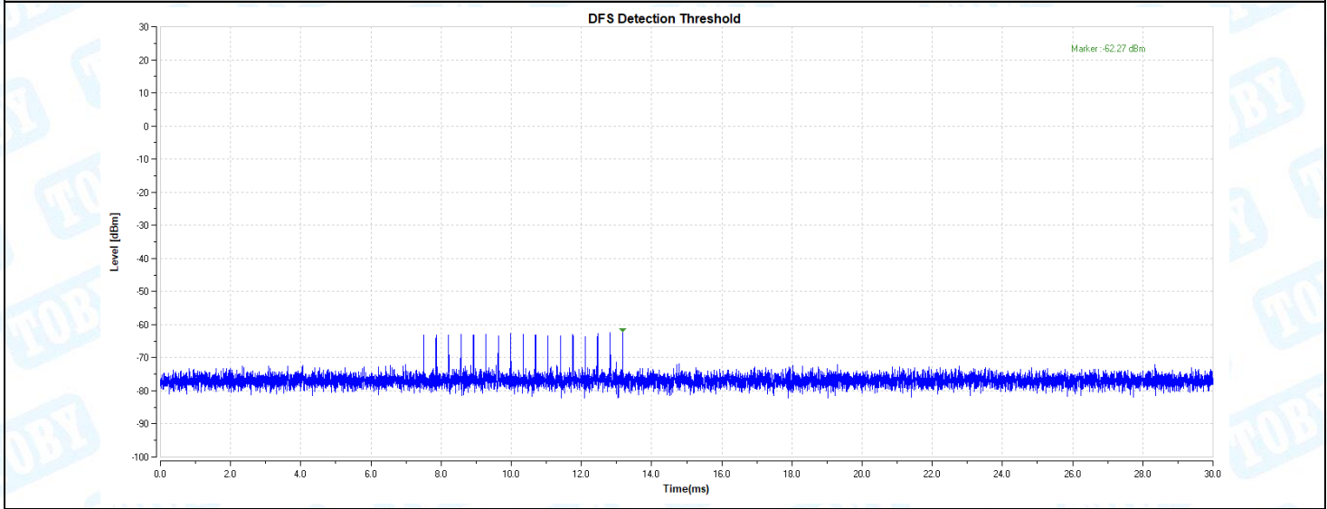
11AX40-5270-Type3-PASS
