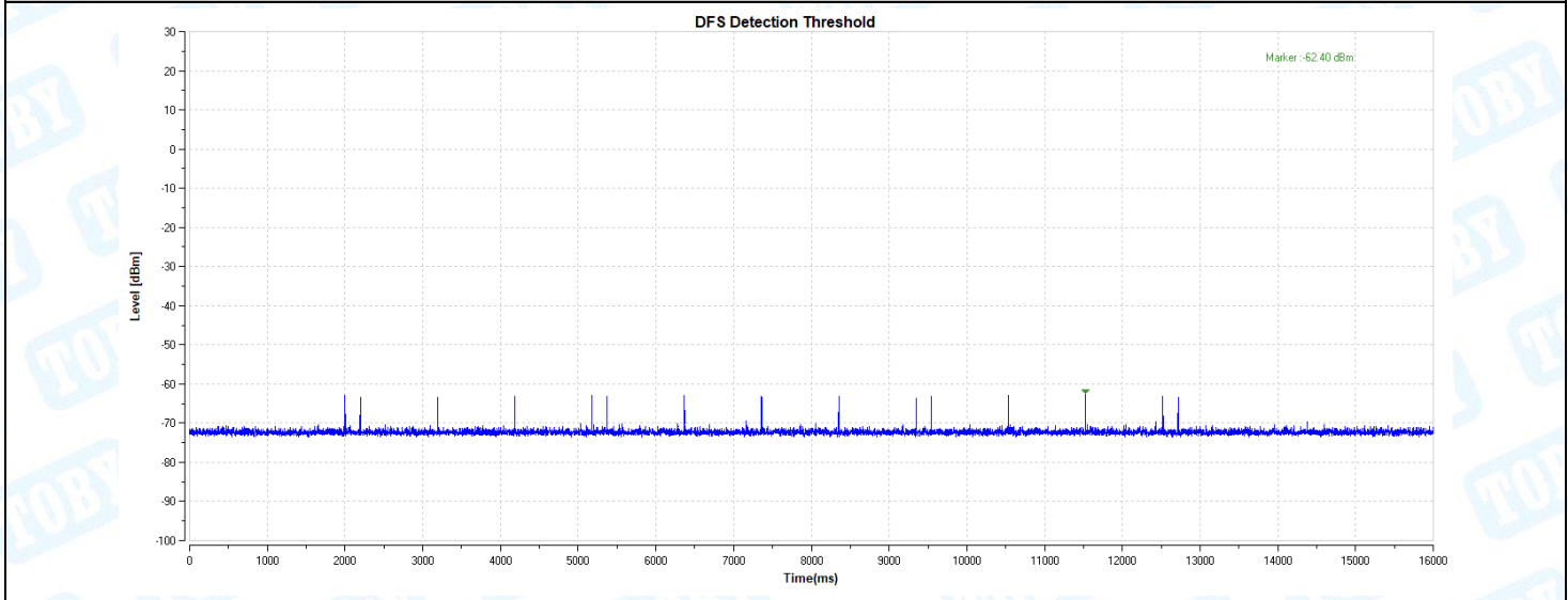
11AX40-5270-Type5-PASS
