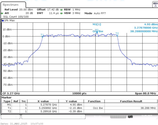
11AX40-5270-PASS
