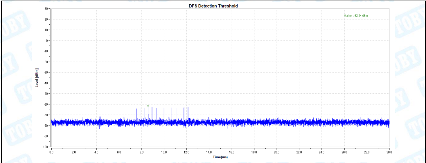
11AX40-5270-Type4-PASS
