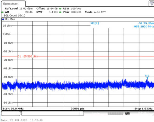
11G-Ant1-2462-30~1000-PASS
