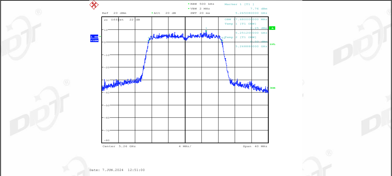
11AC20MIMO_Ant1_5280
