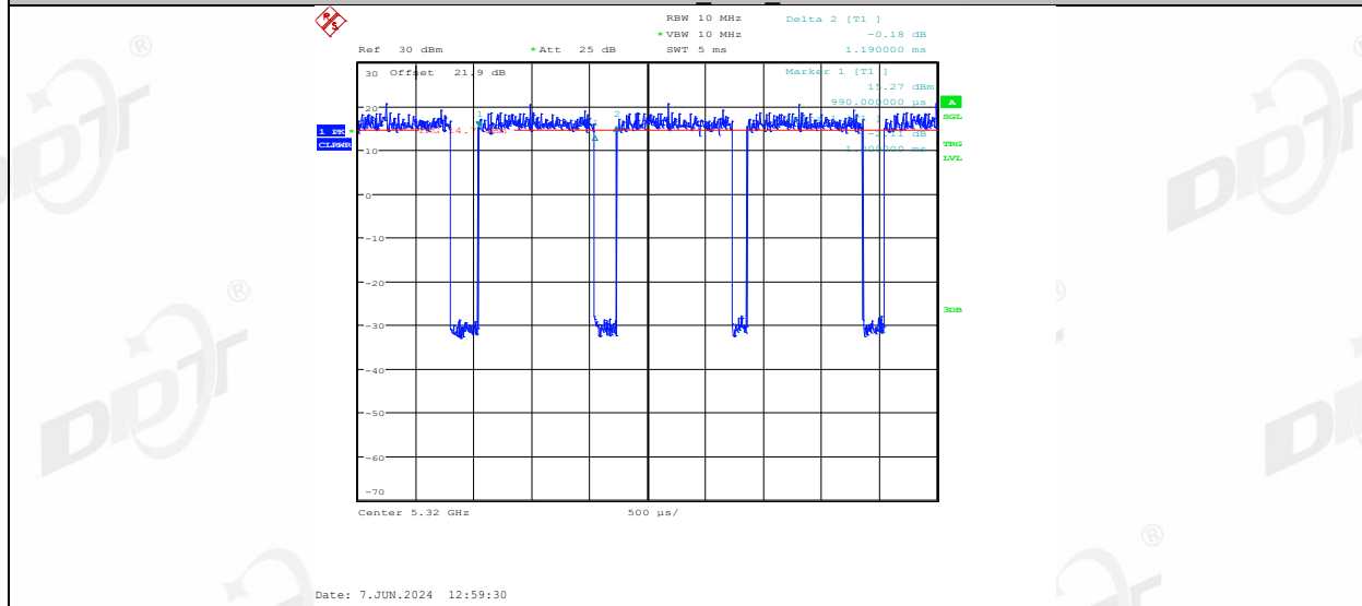
11AC20MIMO_Ant2_5320
