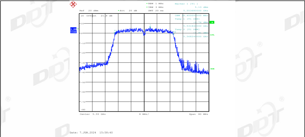
11AC40MIMO_Ant2_5550
