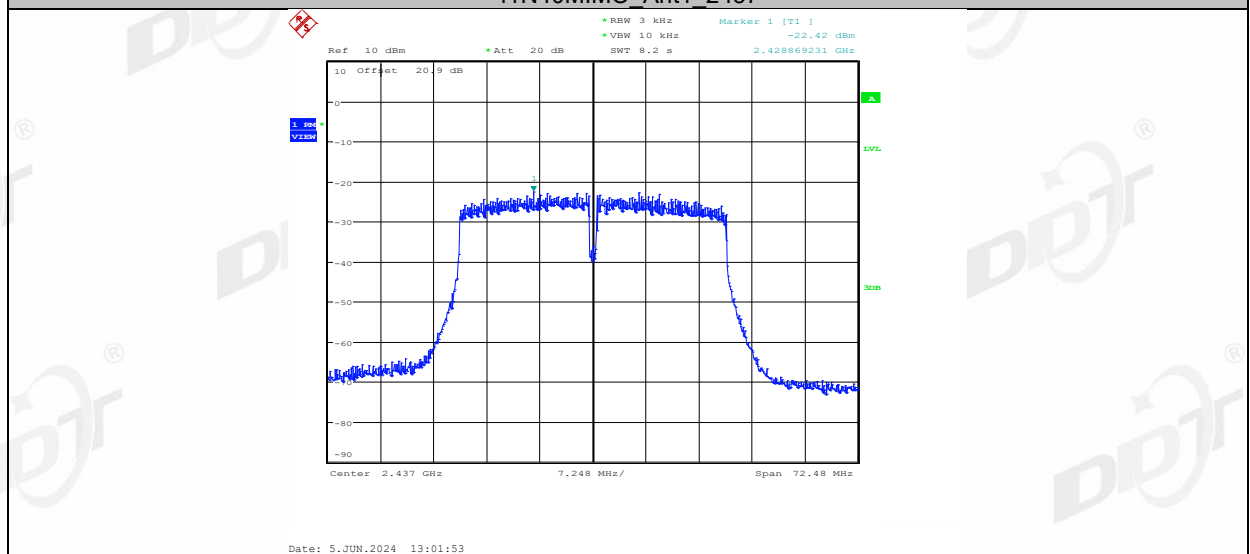
11N40MIMO_Ant2_2437
