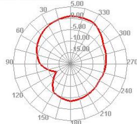
2450.000MHz H
