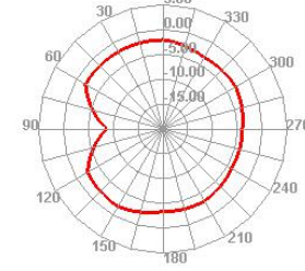
2500.000MHz E2
