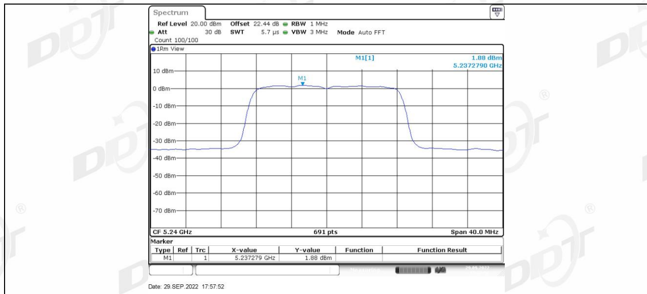
11A_Ant2_5240
