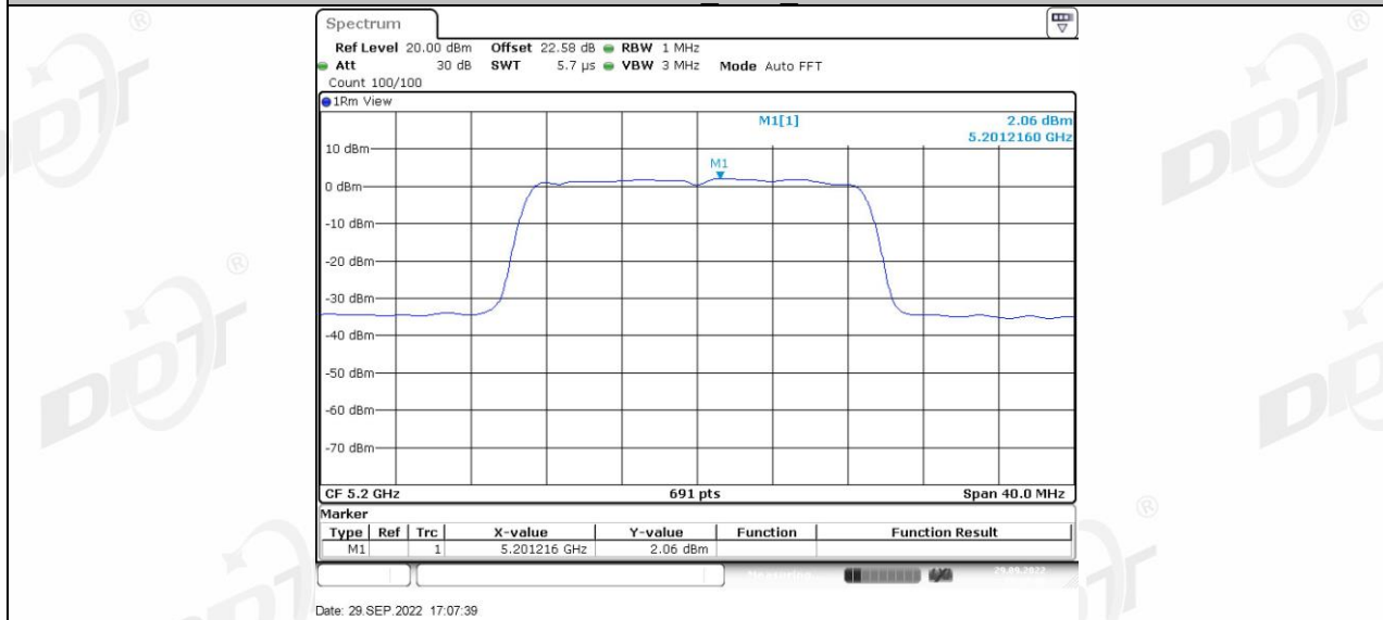
11N20MIMO_Ant2_5200
