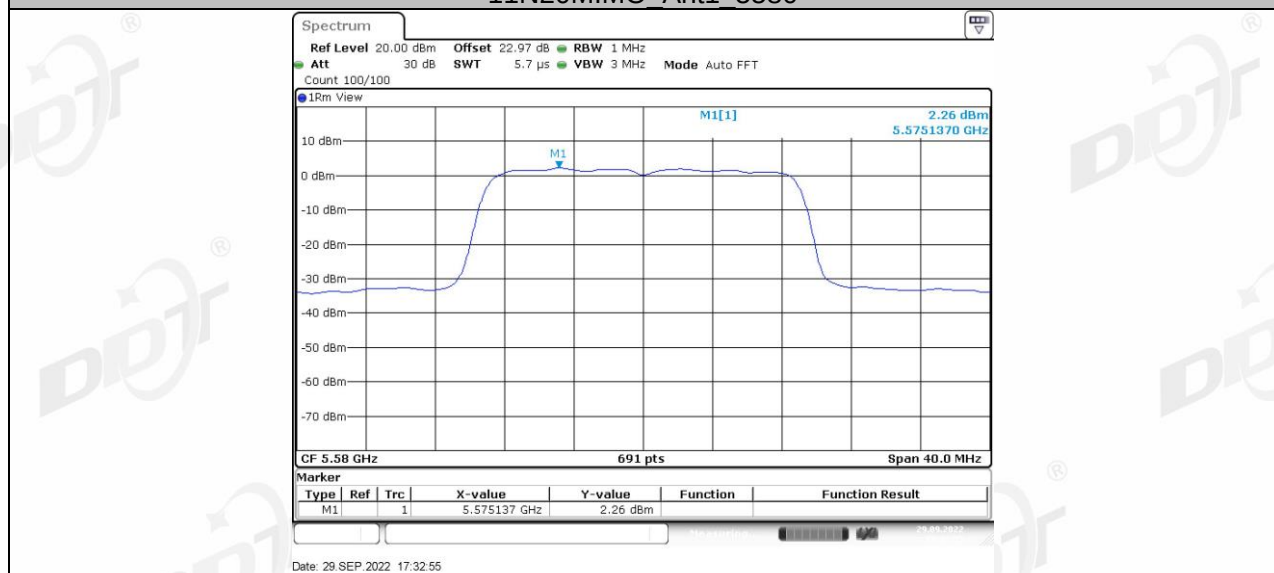
11N20MIMO_Ant2_5580
