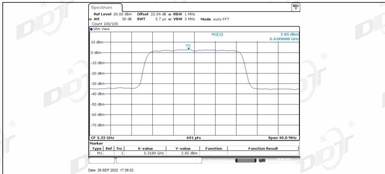
11N20MIMO_Ant2_5320
