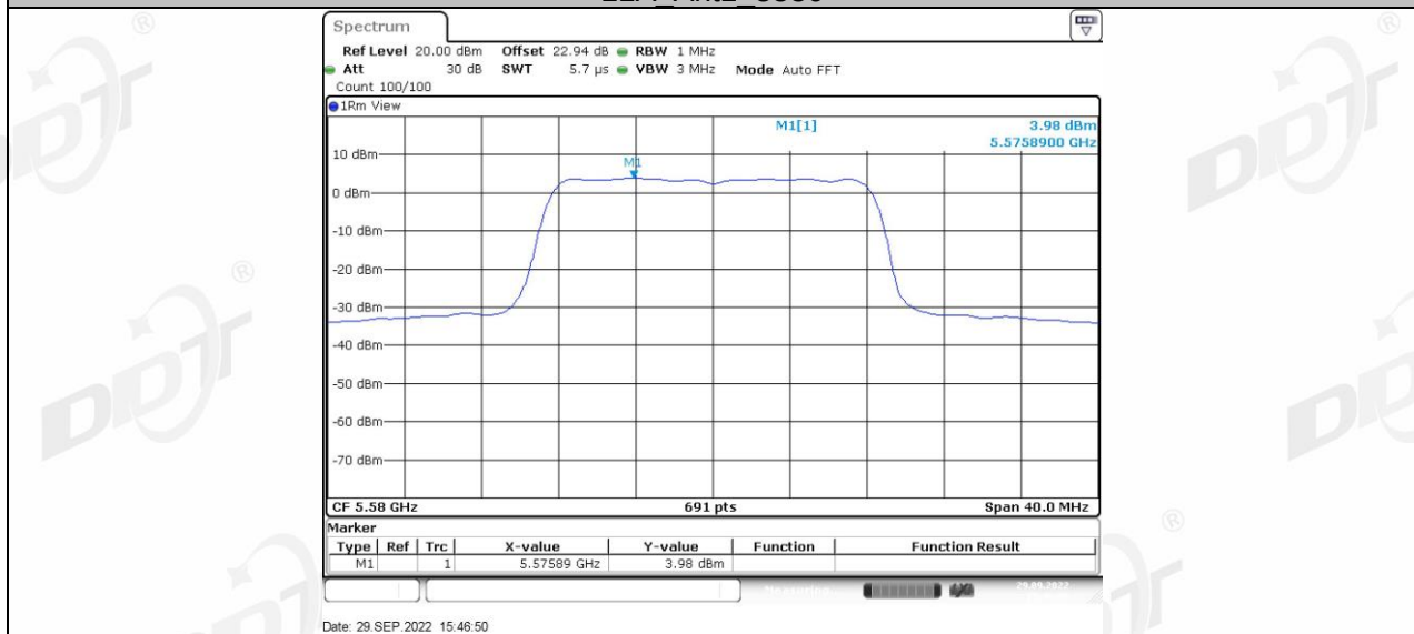
11A_Ant2_5580
