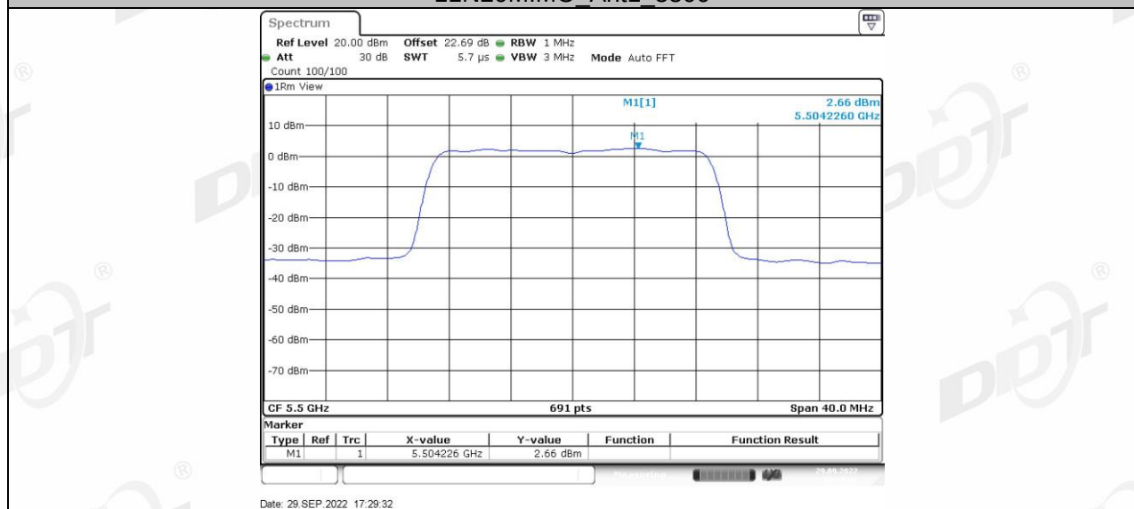
11N20MIMO_Ant2_5500
