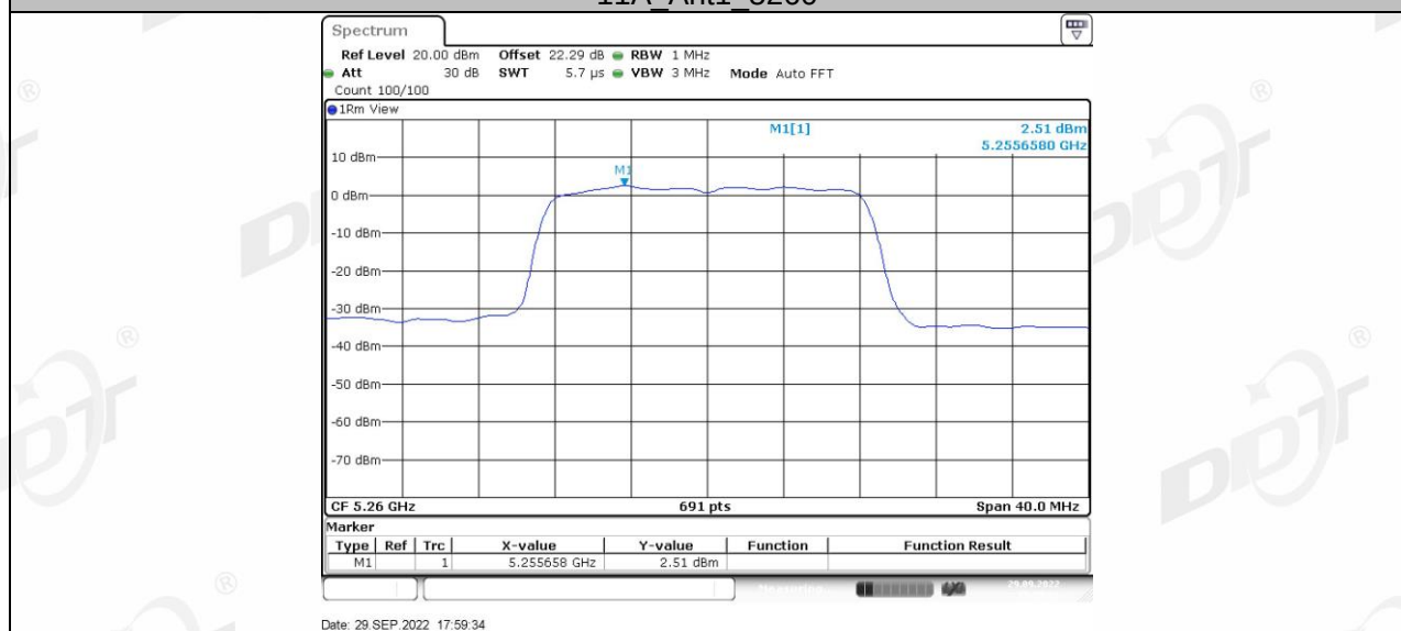
11A_Ant2_5260
