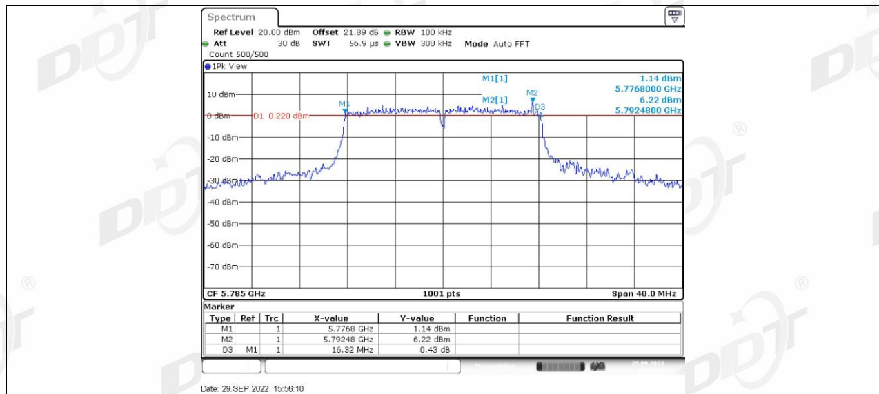
11A_Ant2_5785
