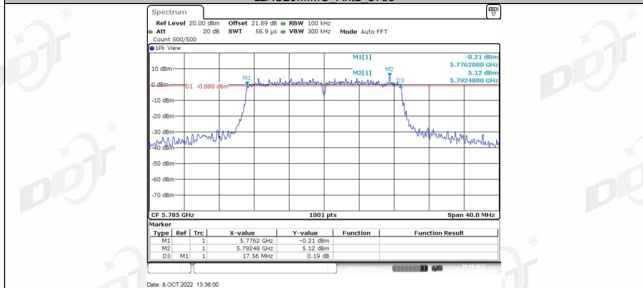
11AC20MIMO_Ant2_5785
