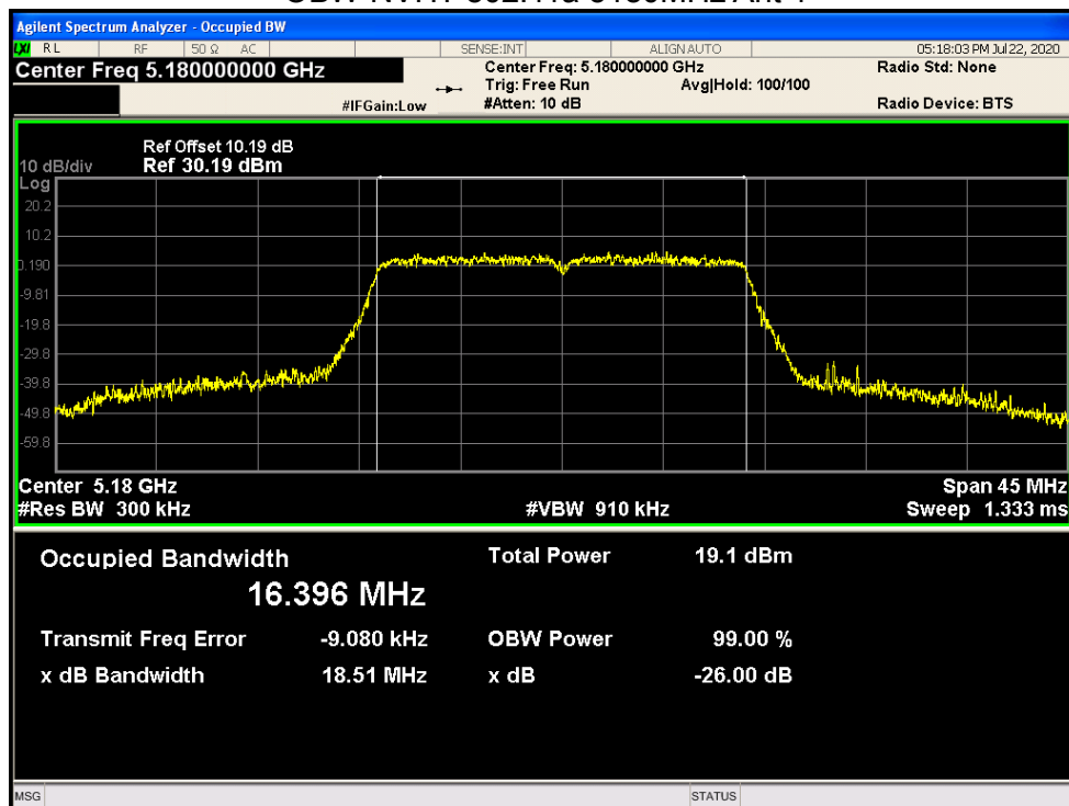
OBW NVHT 802.11a 5180MHz Ant 1
