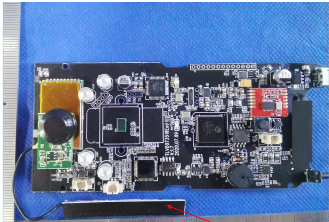
PIFA Antenna
