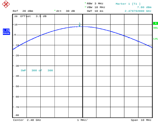
\pi/4 -DQPSK_High 7.80dBm
