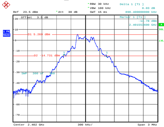
GFSK_Low 0.890MHz
