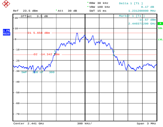
\pi/4 -DQPSK_Middle 1.231MHz
