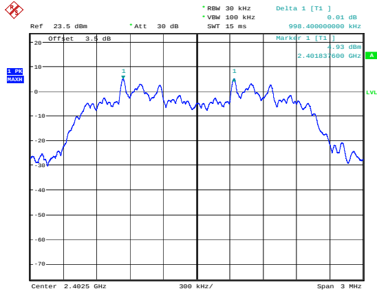
\pi/4 -DQPSK_Low 0.998MHz
