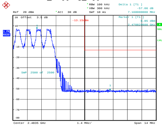
GFSK_Hopping_Upper 57.06dB
