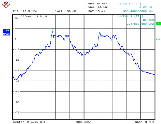
GFSK_High 0.998MHz
