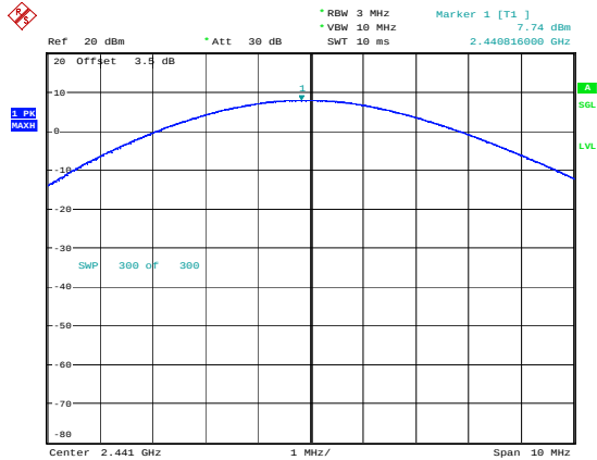
\pi/4 -DQPSK_Middle 7.74dBm
