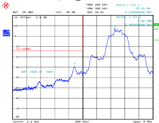
\pi/4 -DQPSK_Low 35.51dB
