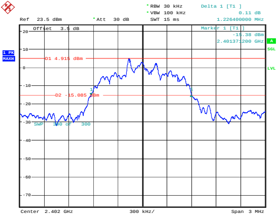
\pi/4 -DQPSK_Low 1.226MHz
