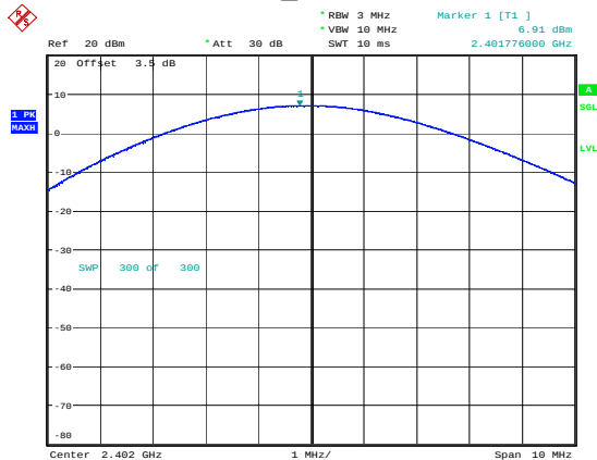
\pi/4 -DQPSK_Low 6.91dBm
