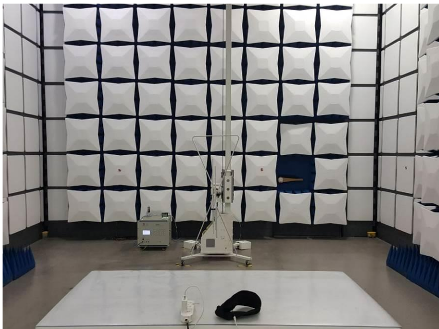
30MHz-1000MHz
