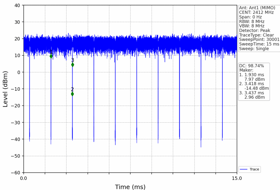
802.11ax(HEW20)_LCH_2412MHz_RU242_Left_Ant1 (MIMO)_NTNV
