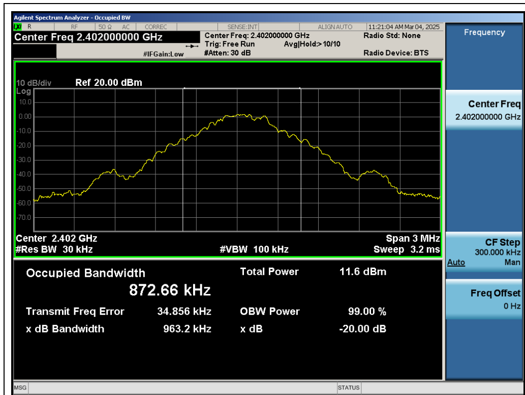
Test_Graph_BR_ANT1_2402_1Mbps_OBW
