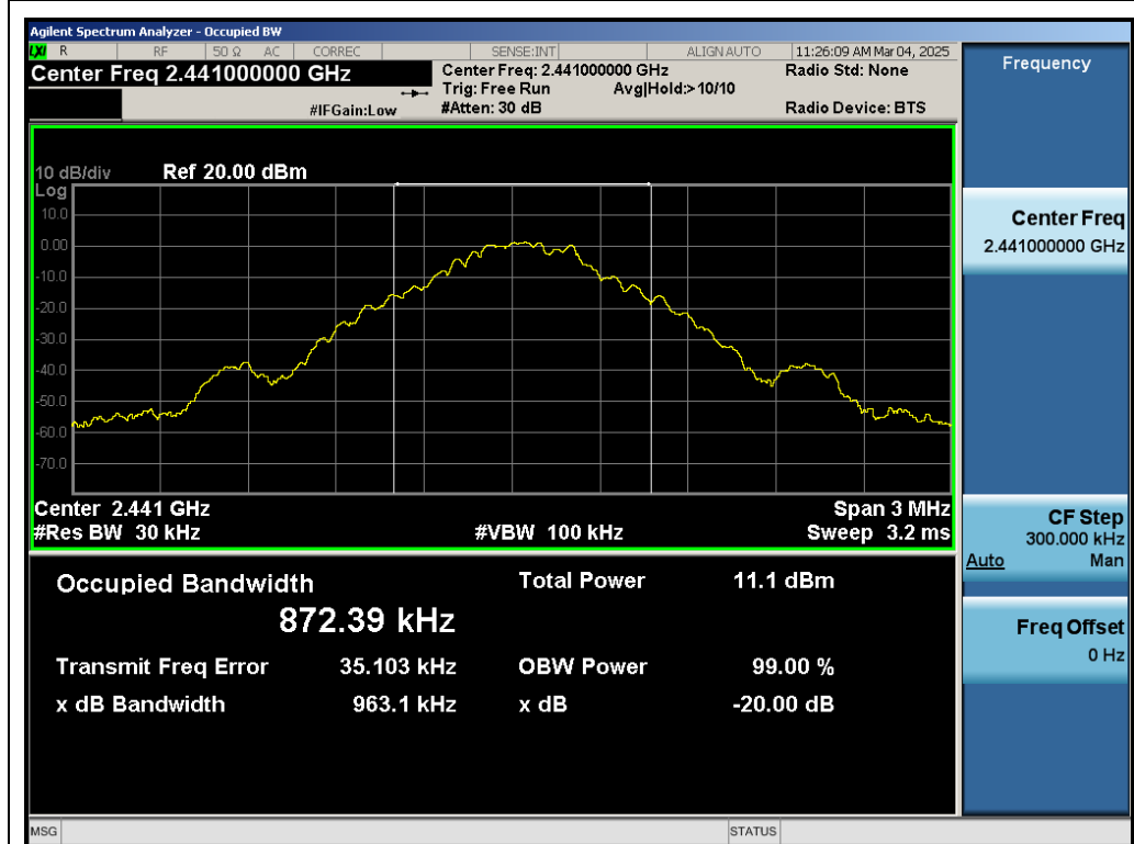
Test_Graph_BR_ANT1_2441_1Mbps_OBW
