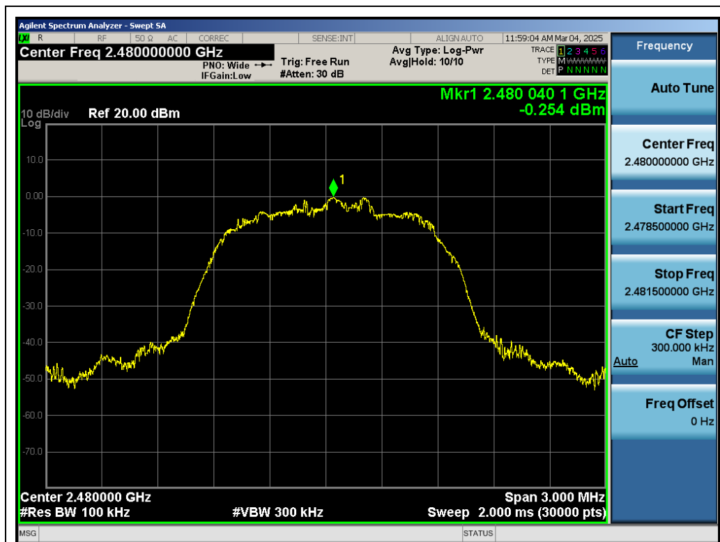
Test_Graph_EDR_ANT1_2480_3Mbps_Reference Level
