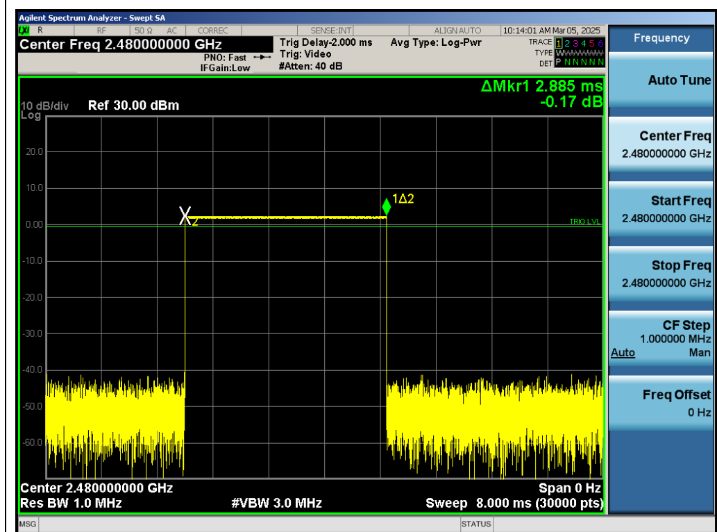
Test_Graph_BR_HOP_ANT1_NA_1Mbps_2480_Time per Burst
