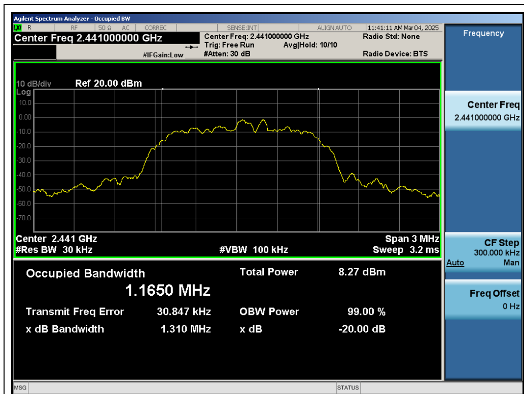
Test_Graph_EDR_ANT1_2441_2Mbps_OBW
