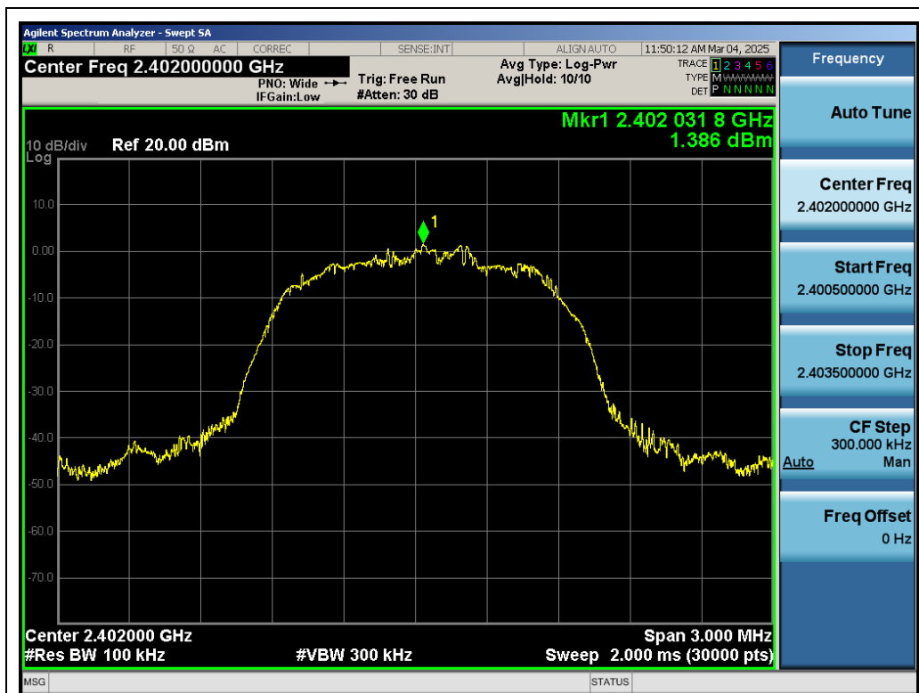
Test_Graph_EDR_ANT1_2402_3Mbps_Reference Level
