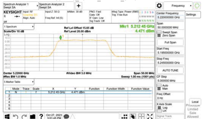
802.11a_20MHz_WLAN2_5220MHz
