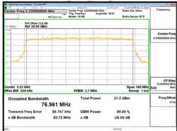
802.11ax_80MHz_Chain1_5530MHz
