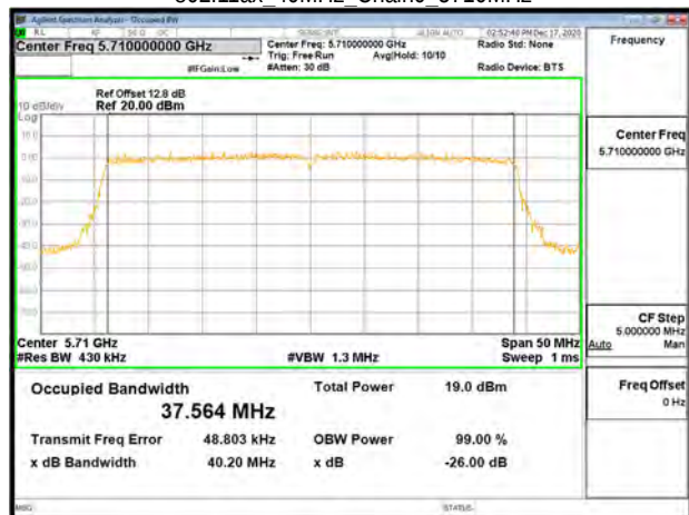
802.11ax_40MHz_Chain0_5710MHz
