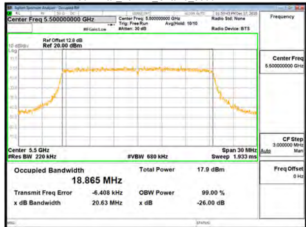
802.11ax_20MHz_Chain0_5500MHz
