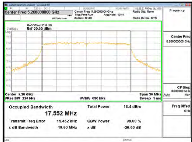
802.11n_20MHz_Chain1_5260MHz
