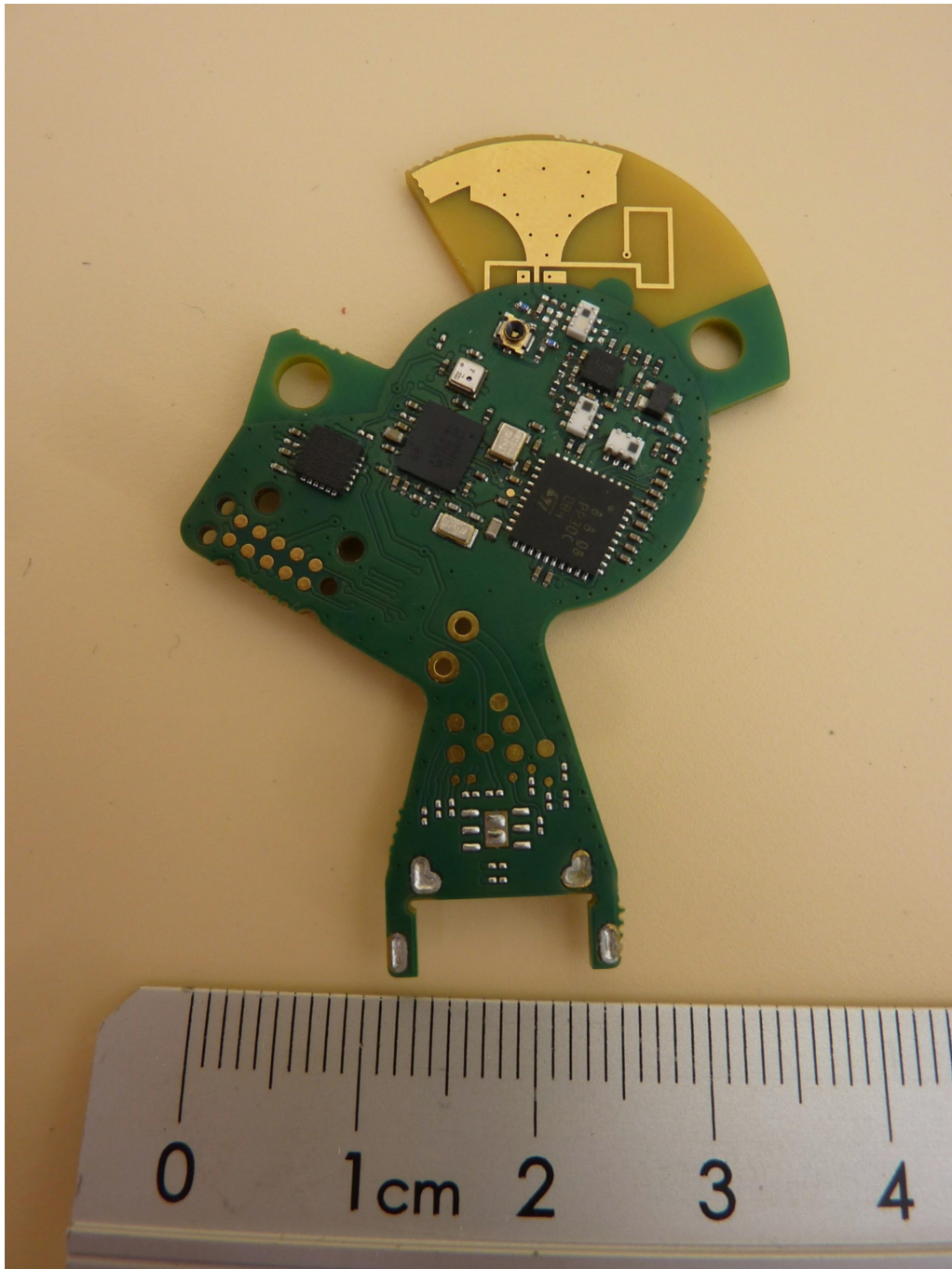
omlox WTag, PCB, bottom view
