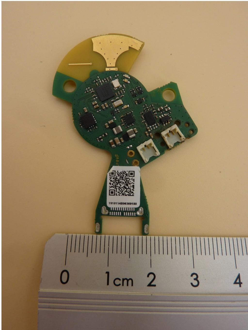
omlox WTag, PCB, top view
