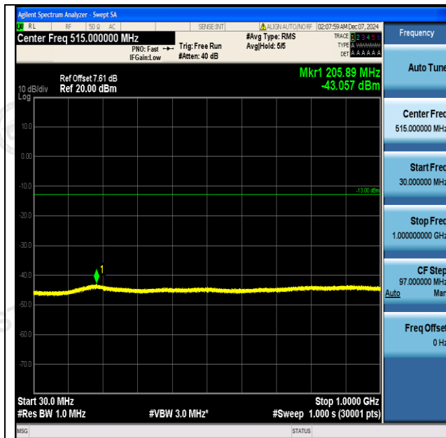
GSM1900-512-0-30~1000MHz-PASS
