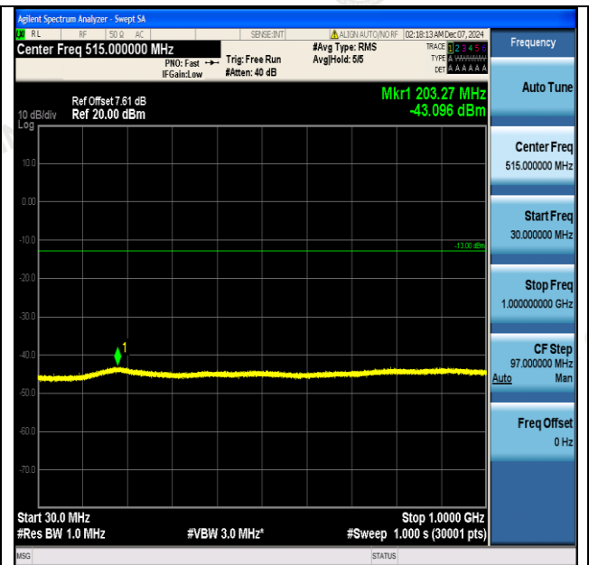
GPRS1900-512-0-30~1000MHz-PASS
