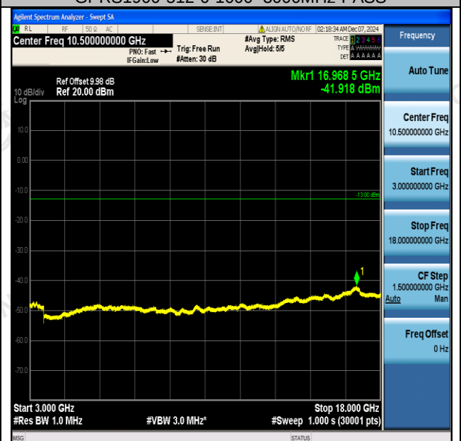
GPRS1900-512-0-3000~18000MHz-PASS
