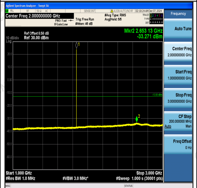
GPRS1900-512-0-1000~3000MHz-PASS
