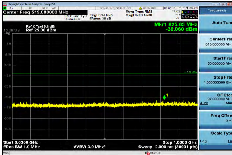
EGPRS1900-810-30~1000
