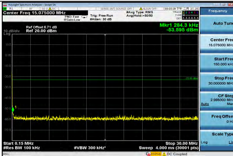
GPRS1900-661-0.15~30
