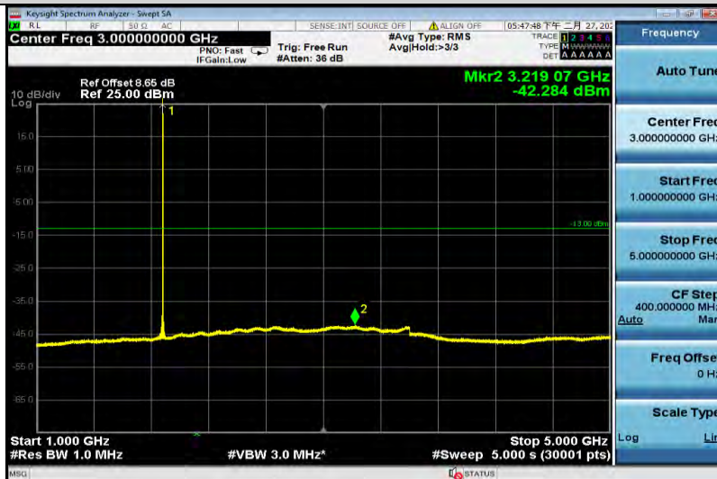
GSM1900-661-1000~5000
