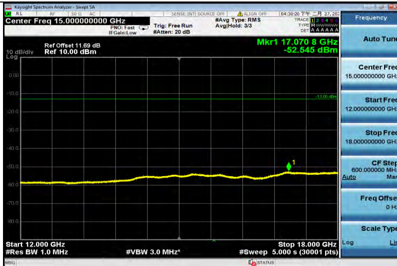
GPRS850-251-12000~18000
