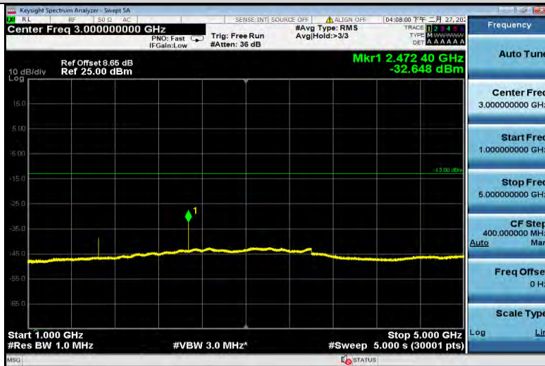
GSM850-128-1000~5000
