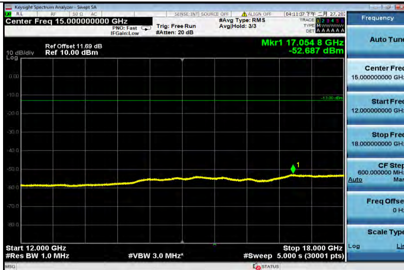
GSM850-251-12000~18000
