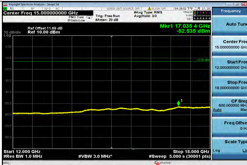
GPRS850-190-12000~18000
