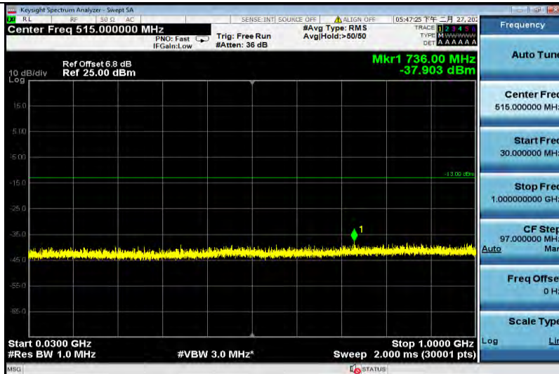
GSM1900-661-30~1000
