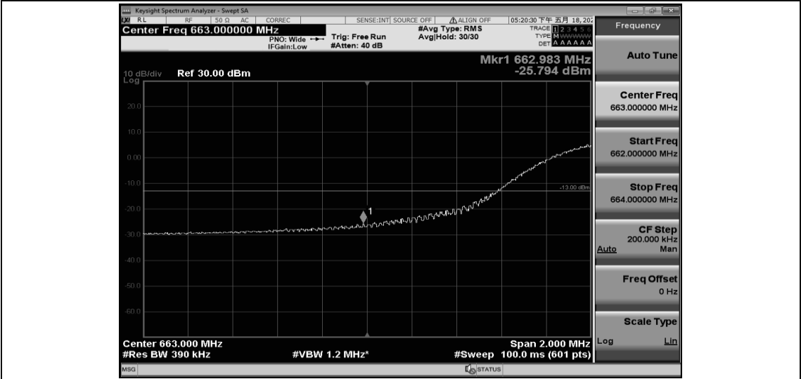
Band71-20MHz-QPSK-133372-100RB#0
